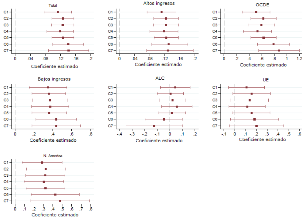
Figura B1: Control de robustez - Cambio de instrumento
