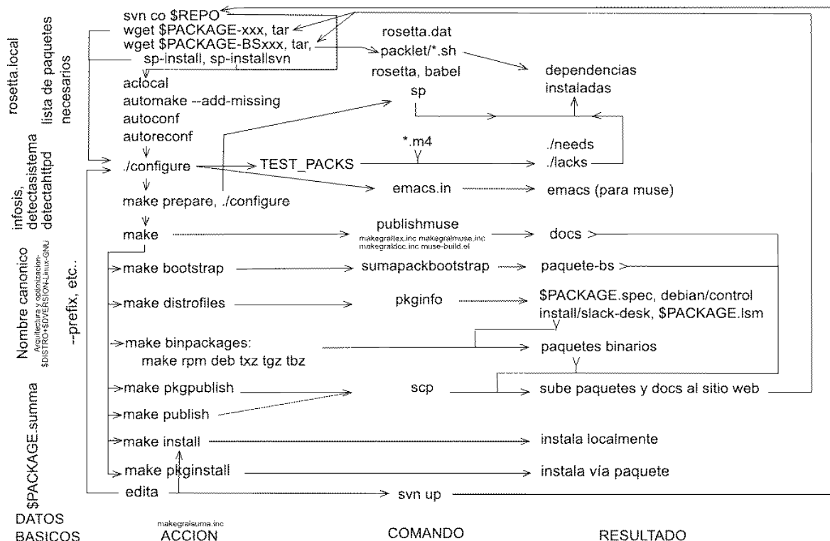
Figura 2: Esquema de autosuma, o el apoyo de Sumapack a las autotools.
