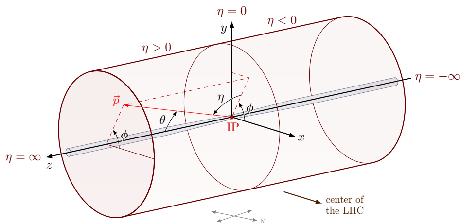
Figura 2.6: Diagrama del sistema de coordenadas del detector ATLAS [61].
