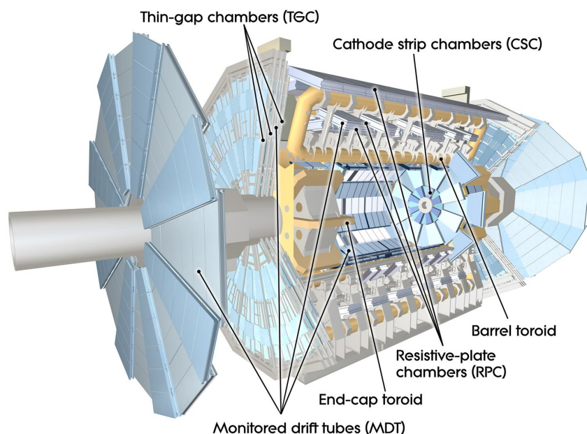
Figura 2.13: Espectrómetro de muones junto con el sistema de imanes toroidales (amarillo) del detector ATLAS [70].
