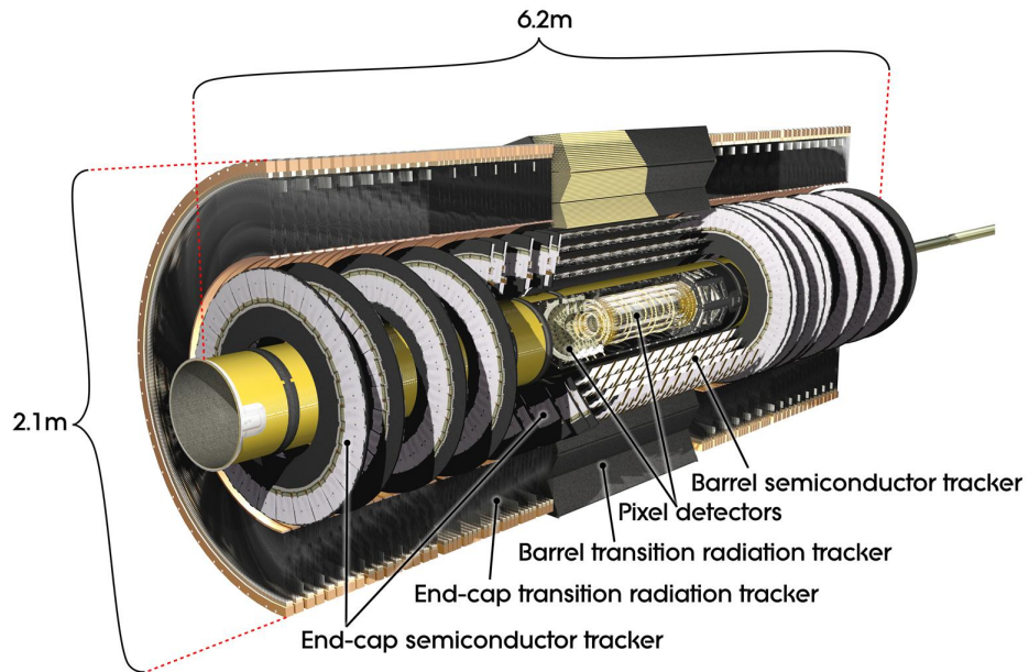
Figura 2.8: Esquema del detector interno de ATLAS, donde se señalan los diferentes módulos [64].
