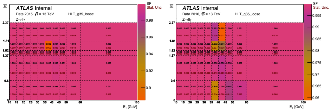
Figura 4.9: Scale Factors para el trigger HLT_g35_loose en función de E_T y \eta con un WP de aislamiento FixedCutTightCaloOnly, para el año 2015 (izquierda) y 2016 (derecha). En rojo las incertezas estadísticas.
