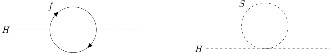
Figura 1.4: Correcciones cuánticas a un loop al parámetro de masa del Higgs m_H^2 debido un fermión de Dirac f (izquierda) y debido un campo escalar S (derecha).
