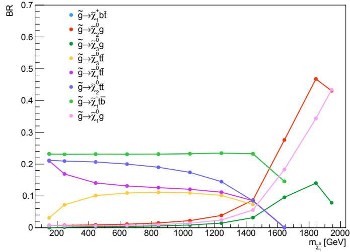
Figura 6.4: Fracción de decaimiento del \tilde{g} con una masa de 2000 GeV en función de la masa del \tilde{\chi}_1^0 .
