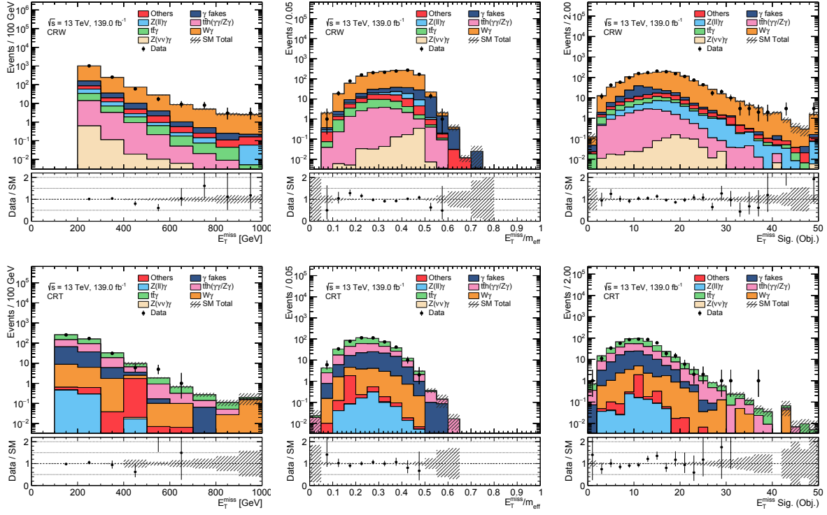
Figura 7.4: Distribuciones preliminares en la región de control CRW y CRT luego del ajuste de solo fondo, para el análisis de producción electrodébil. Las incertezas mostradas son sólo estadísticas.
