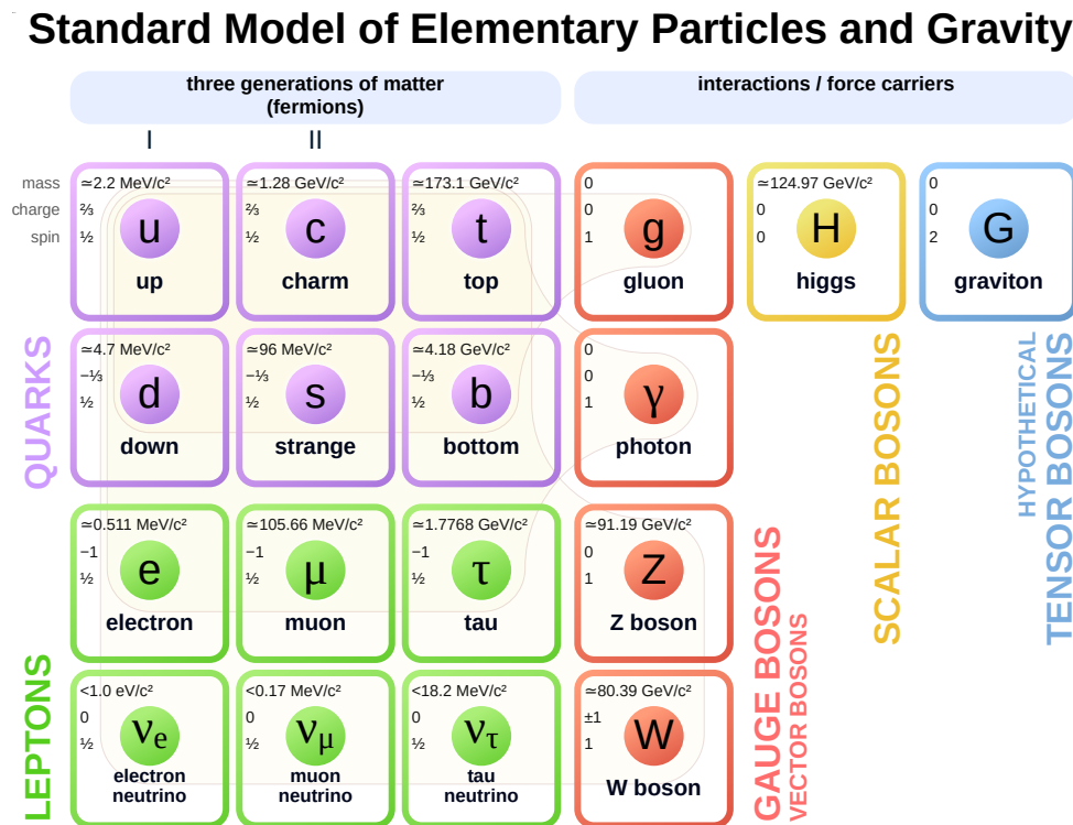
Figura 1.1: Partículas del SM junto con el gravitón. Para cada una se indica su masa, carga eléctrica y spin. Por simplicidad las antipartículas fueron omitidas, y no se hace distinción entre partículas de quiralidad izquierda y derecha.
