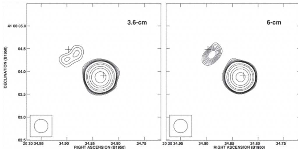
Figura 9: Imágenes tomadas con el Very Large Array. Izquierda: con el receptor centrado en 8 GHz ( \lambda = 3.6 cm). Derecha: con el receptor de 5 GHz ( \lambda = 6 cm) hacia Cyg OB2 #5. La cruz central representa la posición de la binaria cercana O+O, y la cruz a la izquierda, la estrella B terciaria (Contreras et al. 1997). La resolución angular es de ~ 0.3 segundos de arco, como lo indica el círculo en el extremo inferior izquierdo. Contornos: -0.1, 0.1, 0.12, 0.14, ..., 0.24, 0.48, 0.72, 1.44, 2.40, 4.80 y 8.40 mJy/beam (14) .
