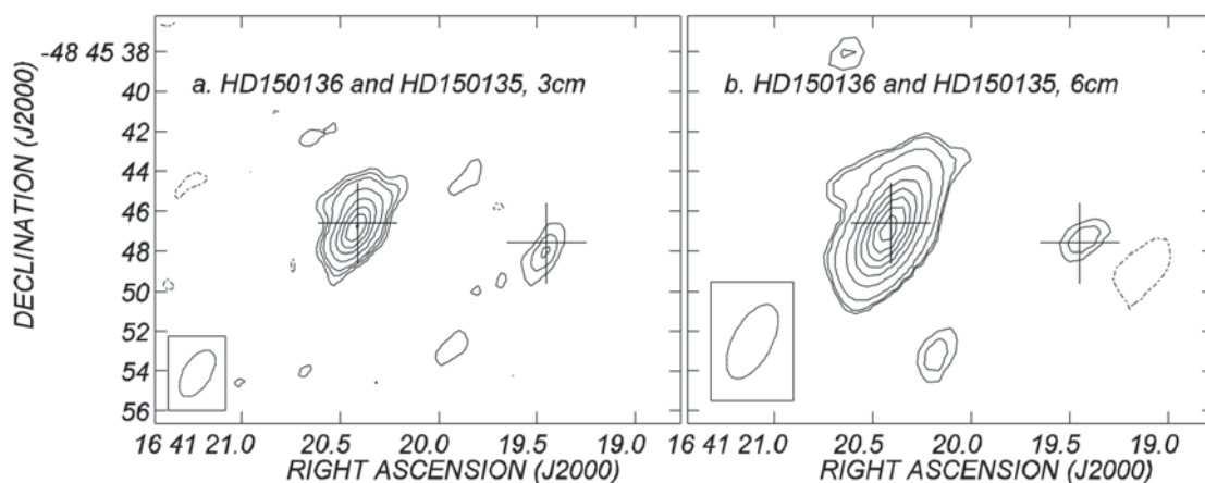
Figura 11: Imágenes tomadas con el Australia Telescope Compact Array hacia las estrellas HD 150135 (cruz derecha) y HD 150136 (cruz izquierda), a) a 8.6 GHz ( \lambda = 3 cm); contornos: -0.08, 0.12, 0.2, 0.3, 0.6, 1.0, 1.4, 1.8 y 2.2 mJy/beam; b) a 4.8 GHz ( \lambda = 6 cm); contornos: -0.15, 0.15, 0.2, 0.4, 1.0, 1.75, 2.5, 3.25, 4.0 y 4.75 mJy/beam.
