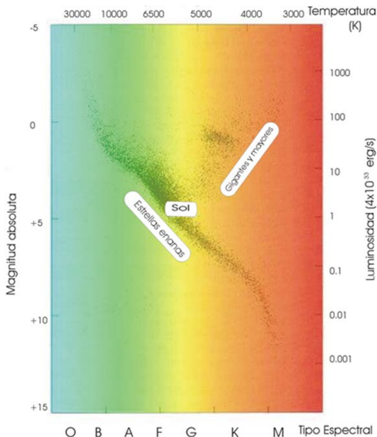
Figura 3: Diagrama Hertzsprung-Russell, donde se ubican las estrellas dependiendo de su brillo intrínseco (magnitud absoluta) y de su temperatura superficial (tipo espectral).
