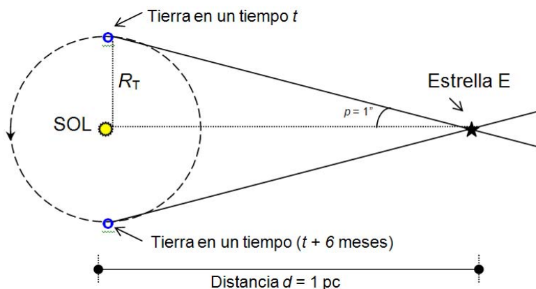
Figura 2: La circunferencia grande de trazos representa aproximadamente la órbita terrestre, de radio R_T . Los círculos pequeños marcan la posición de la Tierra en un tiempo t , y (t + 6 \text{ meses}) = duración del recorrido de media órbita. El círculo estrellado central es el Sol. La estrella negra E es el objeto al que se mide la distancia, proyectada sobre un fondo estacionario como muestran las estrellas grises de la derecha. Cuando el ángulo p , formado por el triángulo de base d y altura R_T , vale 1 segundo de arco (1"), la distancia d a la estrella es de 1 parsec (1 pc).
