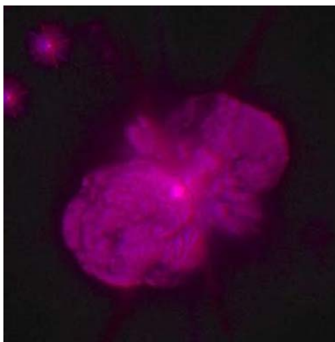
Figura 5: Expansión de gas y polvo a partir de la estrella Eta Carina (HD 93308). Pueden apreciarse los lóbulos y el disco ecuatorial. La imagen fue construida a partir de observaciones separadas en 17 meses, con el Hubble Space Telescope (fuente: J. Morse, C. Davidson y NASA).
