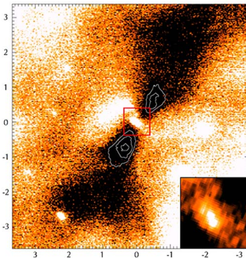
—Figura 13: Imagen en la banda infrarroja Ks, de la silueta de disco obtenida con el telescopio Very Large Telescope, en Paranal, Chile. El disco aparece de color blanco. La región central está ampliada en el extremo inferior derecho (fuente: R. Chini, D. Nurnberger, ESO).
