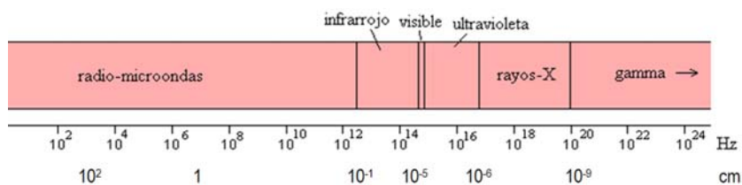
Figura 1: Distintas regiones del espectro electromagnético, en función de la frecuencia (expresada en Hertz o Hz = 1/s), y de la longitud de onda de la radiación (expresada en cm).
