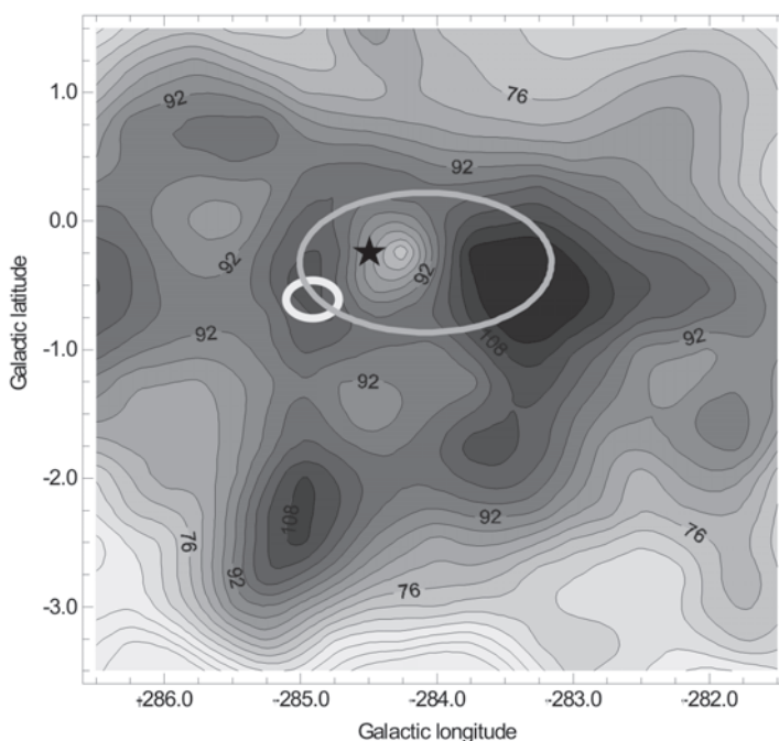
Figura 12: Cantidad de átomos de hidrógeno neutro por \text{cm}^2 (en unidades de 10^{19} ), en la dirección de la línea de la visual, con velocidades del gas entre -21 y -14 km/s. El símbolo estelar marca la posición de Wack 2134. La elipse blanca representa la localización de la fuente de rayos gamma 3EG J1027-5817. La distribución del material alrededor del mínimo que contiene a la estrella estaría formando una especie de cáscara incompleta, o burbuja interestelar, esquematizada por la elipse gris.
