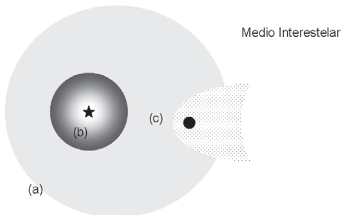
Figura 6: (a), (b) y (c) son las zonas donde se generan frentes de choque, y la consiguiente aceleración de partículas en sistemas estelares binarios. El asterisco representa la estrella primaria, y el punto, la secundaria.
