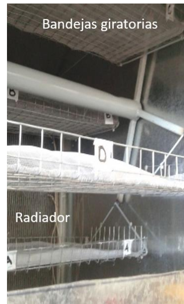
Figura 2 b. Interior de la cabina de secado
