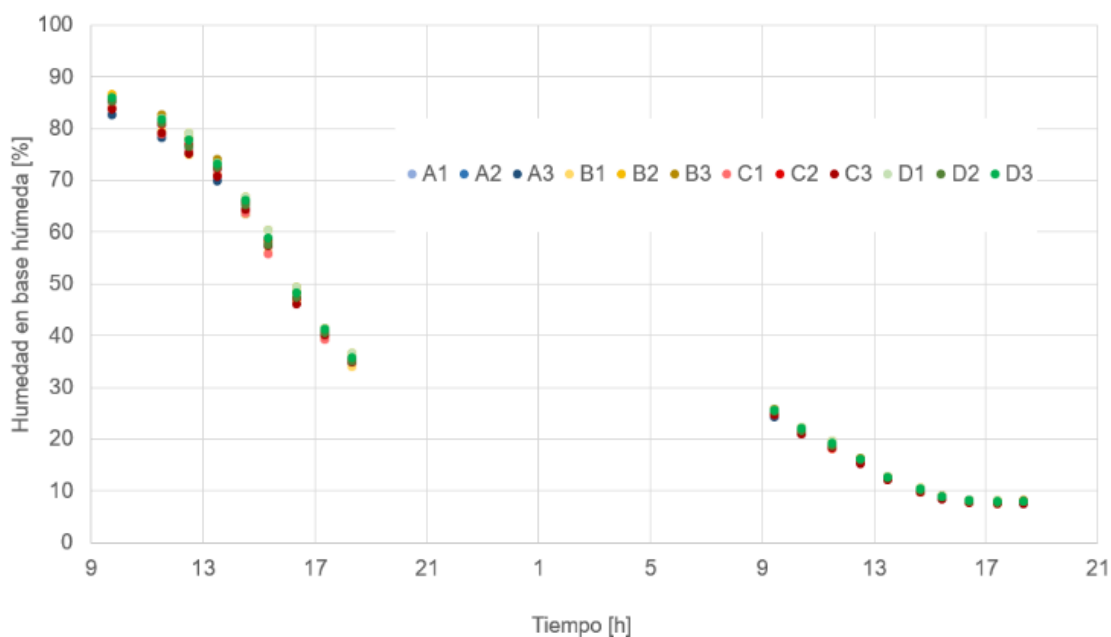
Figura 8. Curva de secado de perejil
