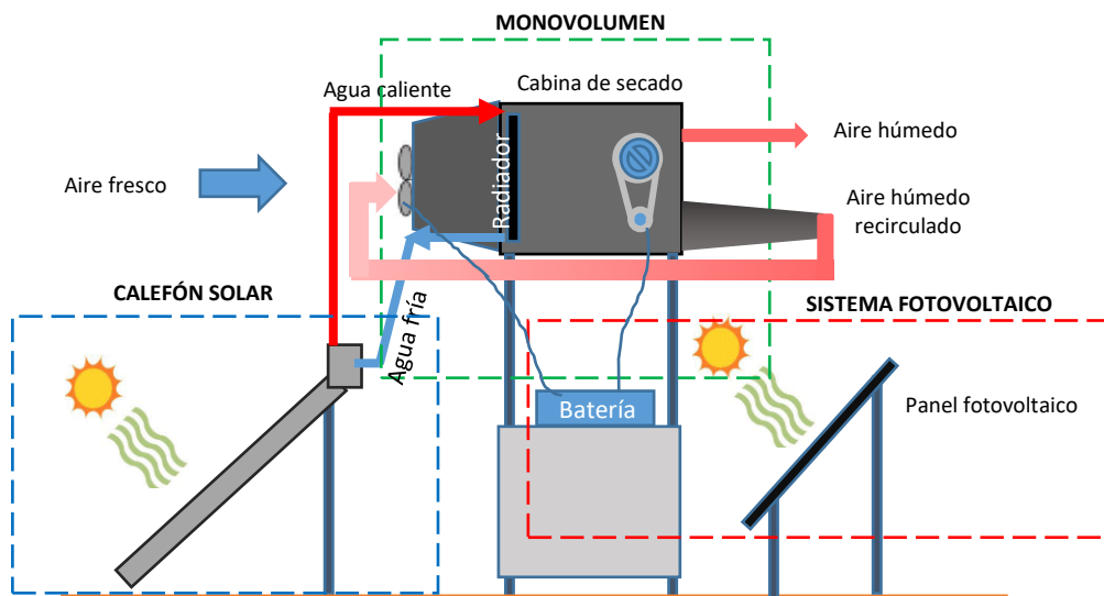
Figura 1. Prototipo de secado solar indirecto con recirculación de aire
