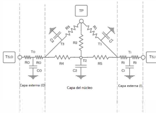
Figura 3: Representación de la capa principal de un APES mediante el modelo RC Combinado.
