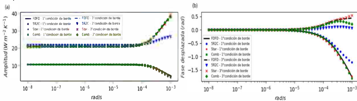
Figura 5: Variación de los perfiles de amplitud y desfase del flujo de calor con respecto a la frecuencia, para la superficie de la pared del tubo.
