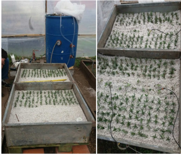
Figura 4: a) Vista del sistema completo en proceso de plantación en el interior del invernadero. b) Sistema completo con las estaquillas plantadas, modulo frontal calefaccionado con sensores en sectores de ingreso y salida del agua caliente, modulo posterior con sustrato frío y sensor de temperatura en el centro.
