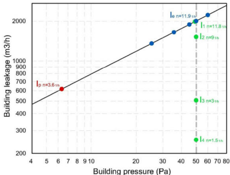
Figura 4: Curva de infiltración de la vivienda. Puntos azules: mediciones obtenidas, a 50 Pa equivalente a 11.9 Vol/h. Punto rojo: infiltración de la vivienda en \text{m}^3/\text{h} a 6.35 Pa, presión de viento promedio para la localidad. Puntos verdes: I1= Vivienda en Albañilería de Ladrillo chilena, I2= Vivienda de hormigón, I3= Valor máximo de infiltración normado para una vivienda c/ventilación natural en Alemania y Austria, I4= Valor máximo de infiltración normado para una vivienda c/ventilación mecánica en Alemania y Austria.
