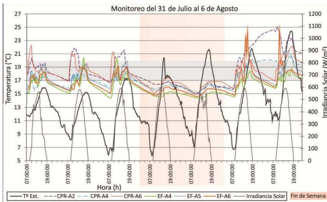
Figura 2. Temperatura e irradiancia solar, evolución temporal. Semana 1 - Invierno.
