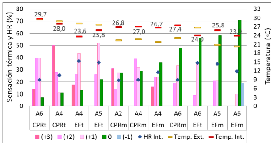
Figura 10: Voto de sensación térmica, en relación a la T^{\circ} y HR interior, y T^{\circ} exterior. Primavera.
