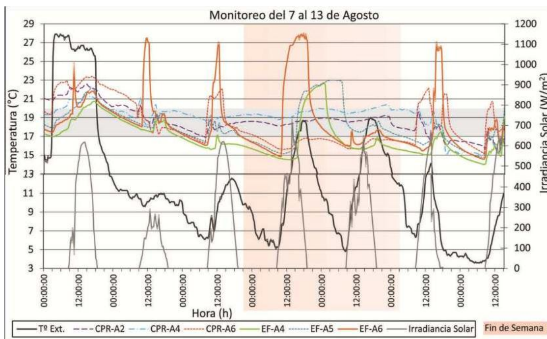
Figura 3. Temperatura e irradiancia solar, evolución temporal. Semana 2 - Invierno.
