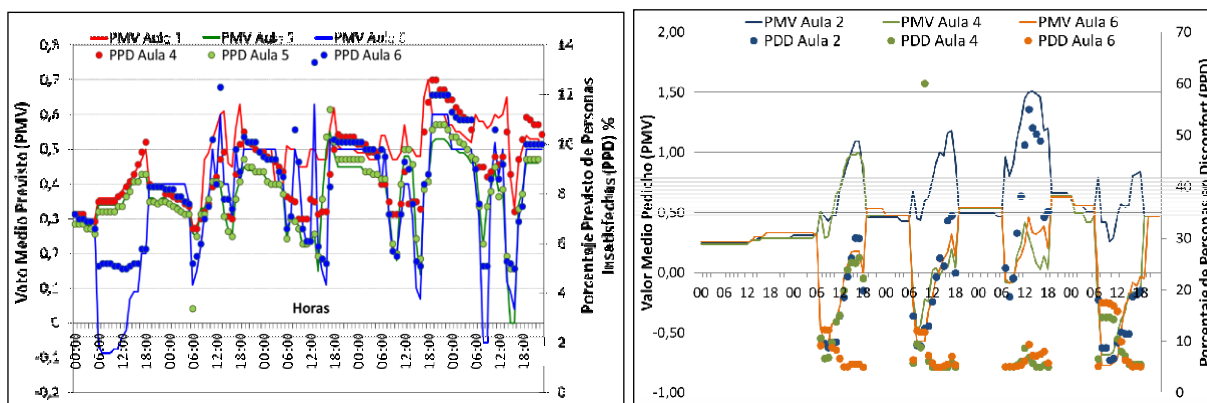
Figura 7: PMV y PPD en Período 2. Izquierda: Caso EF. Derecha: Caso CPR
