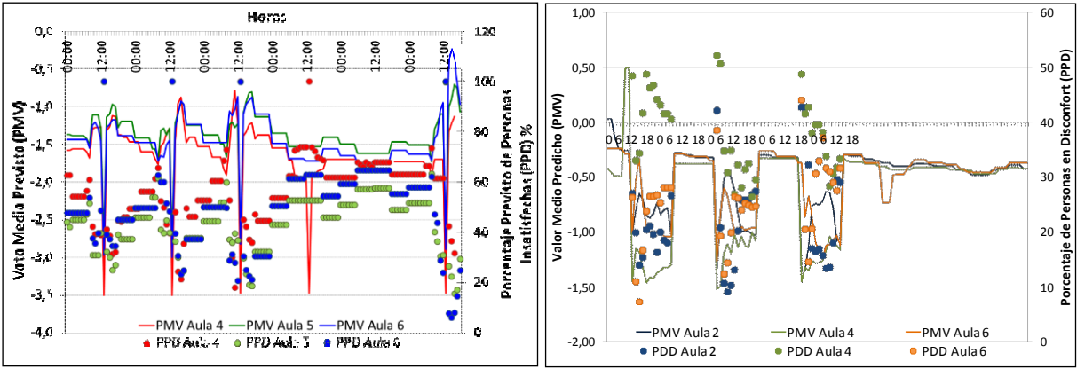
Figura 6: PMV y PPD en Periodo 1. Izquierda: Caso EF. Derecha: Caso CPR
