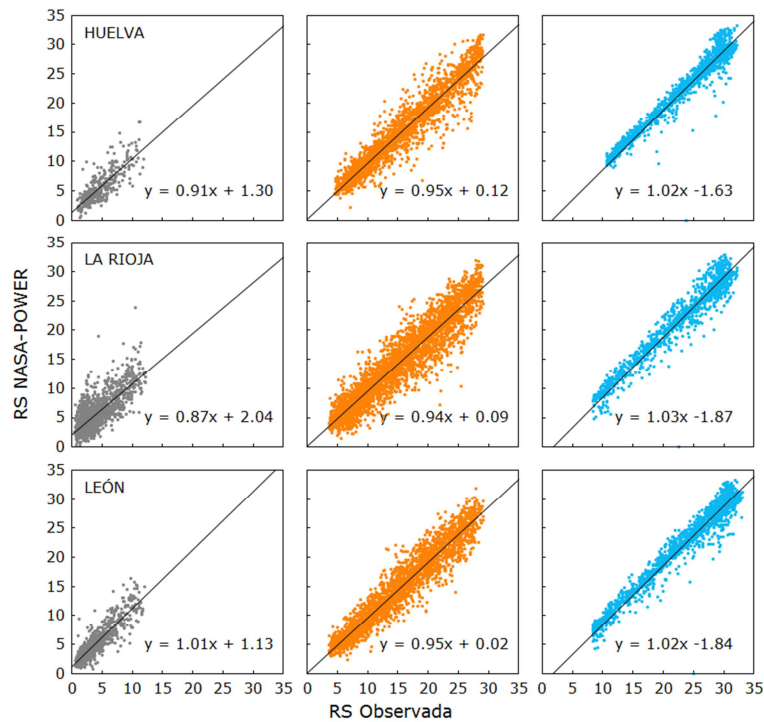
Figura 3: Gráfico de dispersión entre la radiación solar registrada y estimada por NASA-POWER según índice de claridad, para las provincias de Huelva, La Rioja y León (En gris los días nubosos, en naranja los días parcialmente nubosos y en celeste los días claros).
