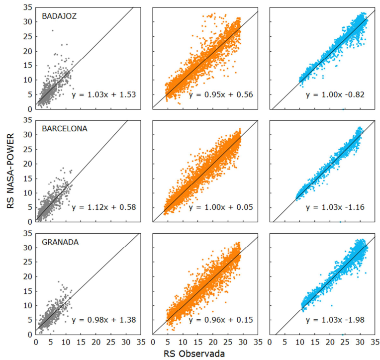
Figura 2: Gráfico de dispersión entre la radiación solar registrada y estimada por NASA-POWER según índice de claridad, para las provincias de Badajoz, Barcelona y Granada (En gris los días nubosos, en naranja los días parcialmente nubosos y en celeste los días claros).
