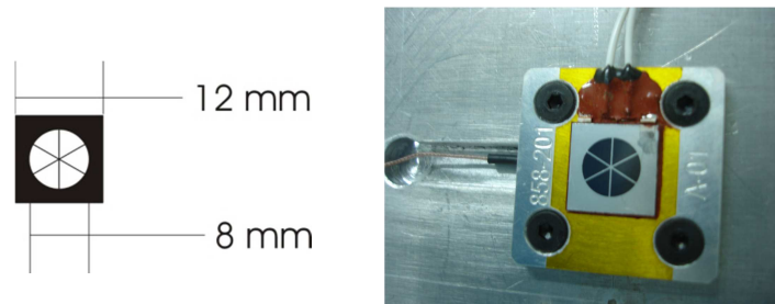
Figura 1: Diseño del CSS (izquierda) y el sensor elaborado (derecha).
