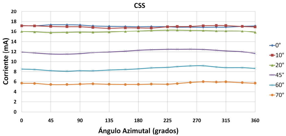
Figura 6: Comportamiento de simetría del CSS.
