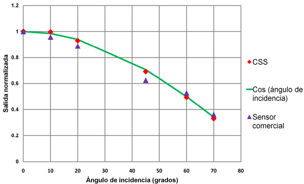
Figura 4: Comparación de la respuesta angular.
