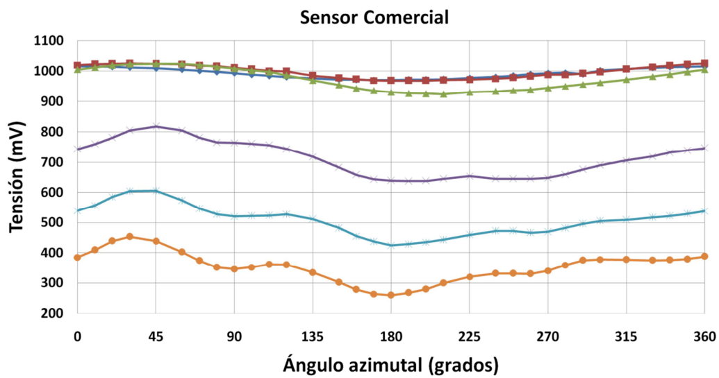
Figura 7: Comportamiento de simetría del sensor comercial.
