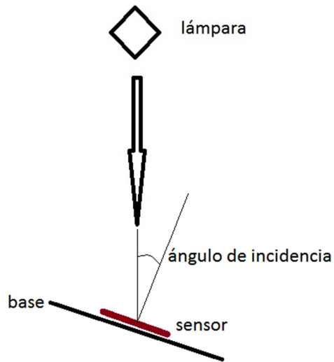
Figura 3: Esquema de medición de la respuesta angular.
