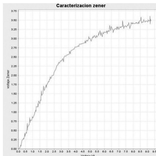
Figura 11. Señal Caracterización Diodo Zener
