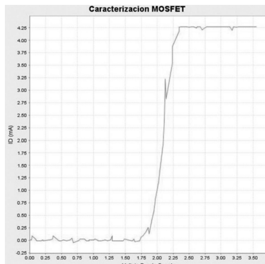
Figura 10. Señal Caracterización Mosfet
