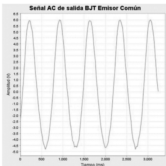
Figura 8. Señal AC Circuito Emisor Común BJT
