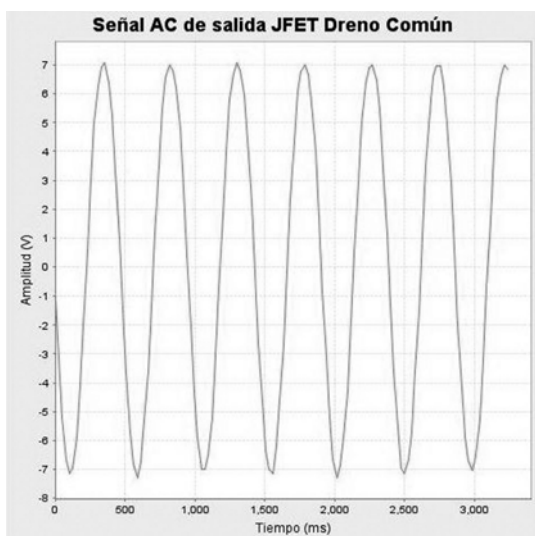
Figura 9. Señal AC Circuito Dreno Común JFET
