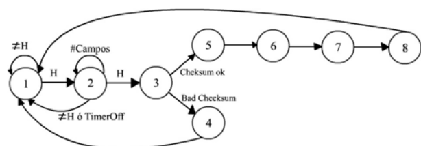
Figura 5. Máquina de estados del microcontrolador
