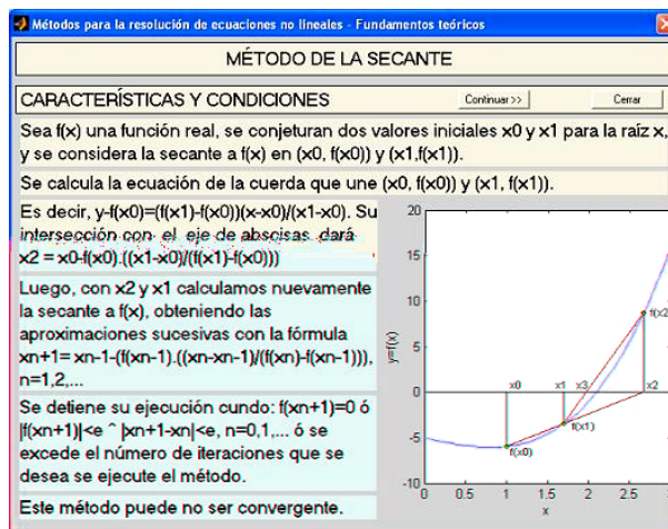
Figura 5. Ayuda teórica sobre el funcionamiento del método de la secante
