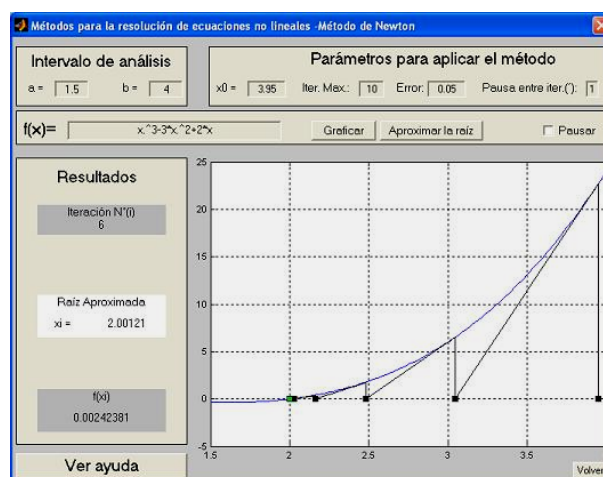
Figura 2. Se muestra la pantalla de la implementación del método de Newton
