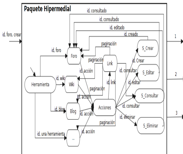
Figura. 2. Modelo DEVS del Paquete Hipermedial.
