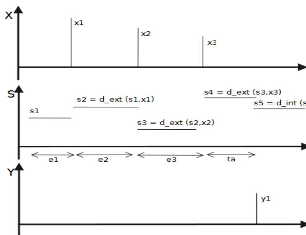
Figura. 3. Gráfico de trayectorias del Modelo DEVS del Paquete Hipermedial.
