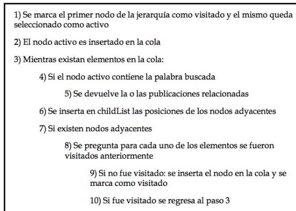
Figura 20. Funcionamiento del algoritmo
