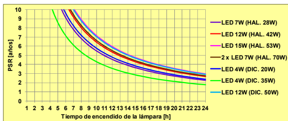
Figura 12. PSR de las lámparas LED's. Tarifa con subsidio.
