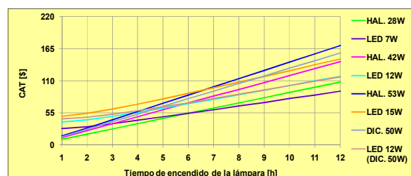
Figura 17. CAT de las lámparas LED's. Tarifa sin subsidio
