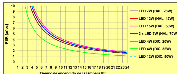
Figura 13. PSR de las lámparas LED's. Tarifa sin subsidio
