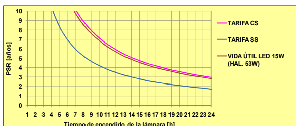
Figura 14. Vida útil y amortización, lámpara LED 15W
