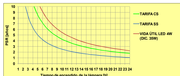
Figura 15. Vida útil y amortización, lámpara LED 4W
