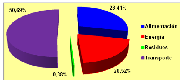
Figura 10. Huellas de CO 2 para Argentina
