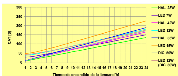
Figura 16. CAT de las lámparas LED's. Tarifa con subsidio
