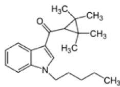
I.6- UR122 (ciclopropil-indol)
