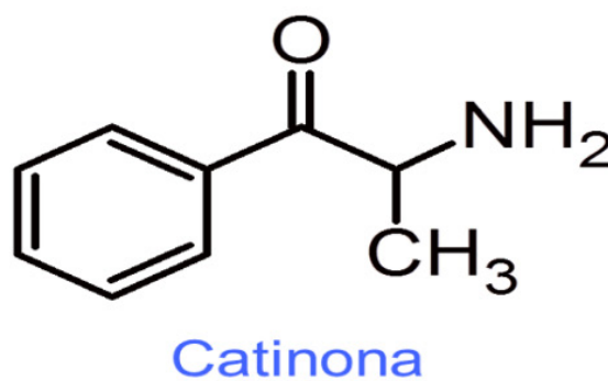
Figura 6: Planta de Kath y estructura del componente principal: catinona.
