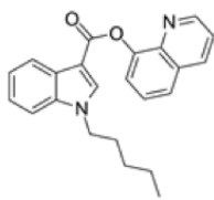
I.5- PB-22 -quinolinil-indol (QUPIC)
