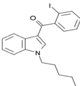
I. 3- AM679 (benzoilindole)
