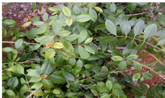
Figura 6: Planta de Kath y estructura del componente principal: catinona.
