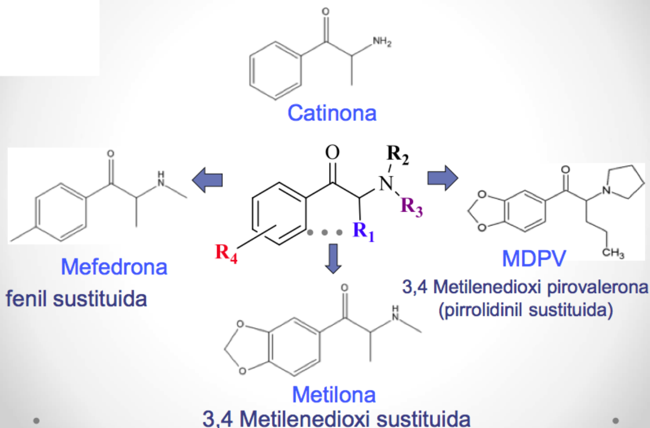
Figura 8: Primera generación de catínonas sustituidas, por sustitución en R1, R2, R3 y R4 (Huestis, 2014).
