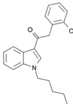
I. 2- JWH 204 (-fenilacetil)
