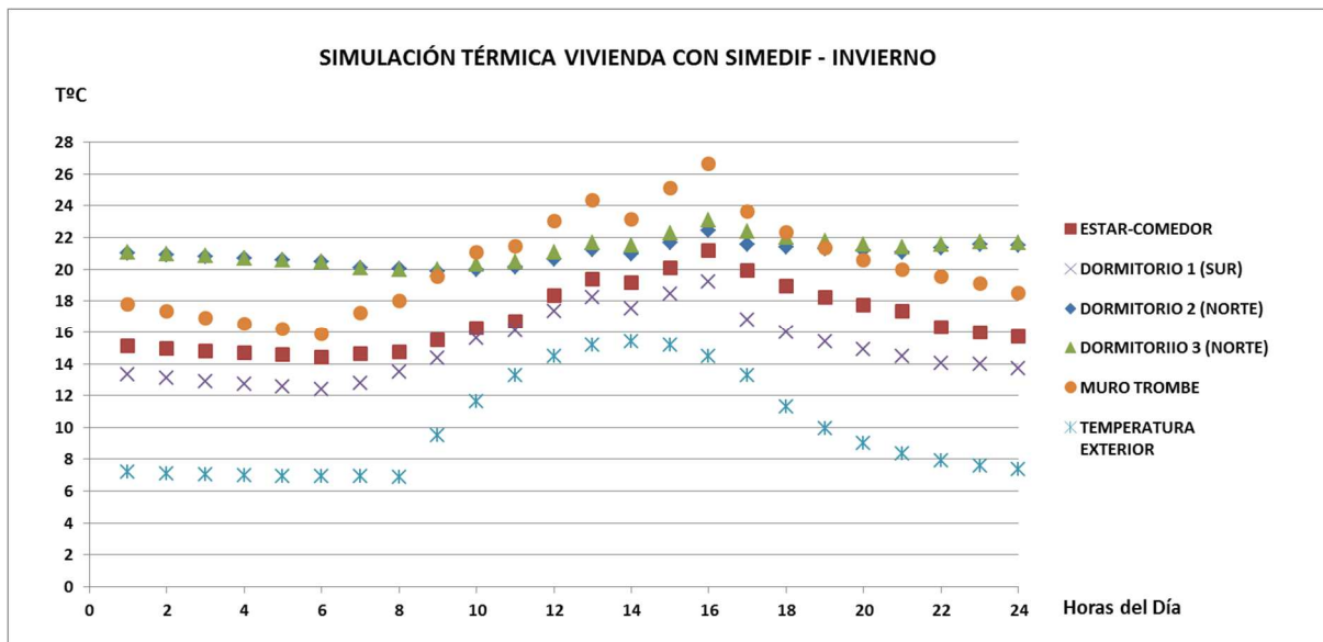
Figura 5: Temperaturas de locales habitables las 24 horas (HSV), del día 13 de julio
