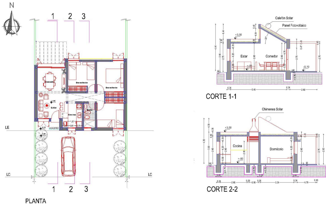
Figura 3: Planta; Corte 1-1 (Estar Comedor) y Corte 2-2 (Cocina y Dormitorio)
