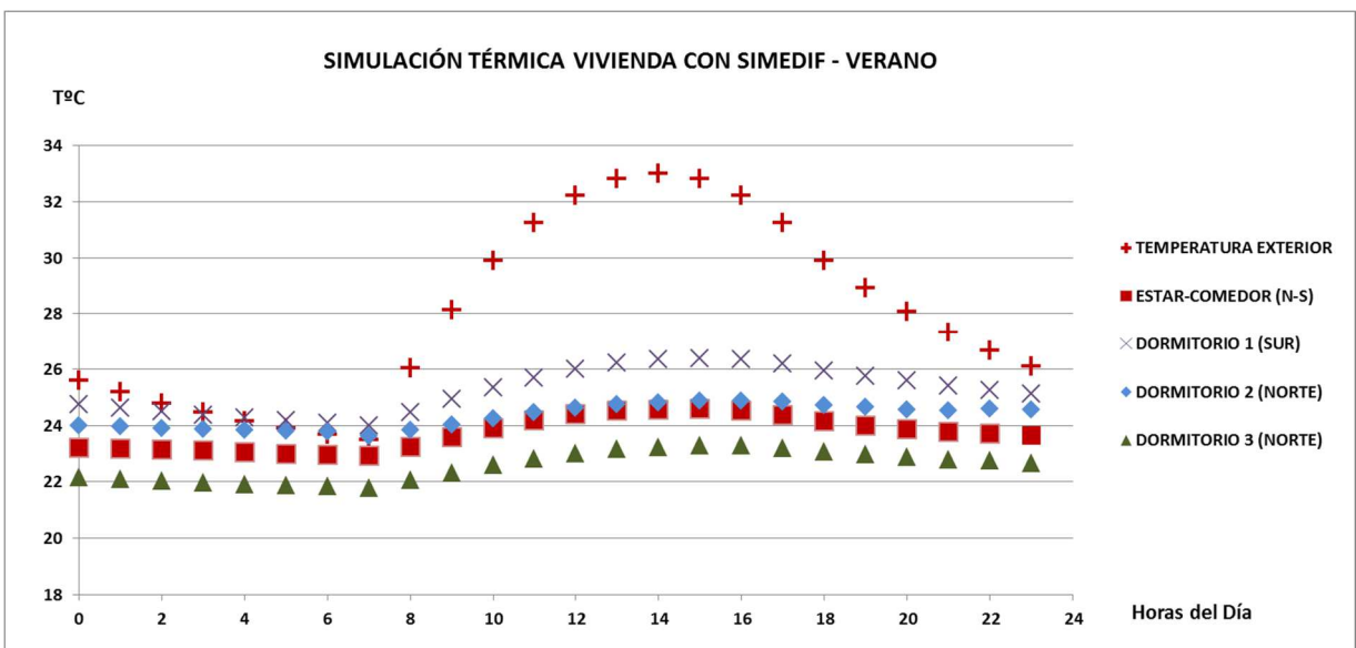
Figura 6: Temperaturas de locales habitables las 24 horas (HSV), del día 15 de enero
