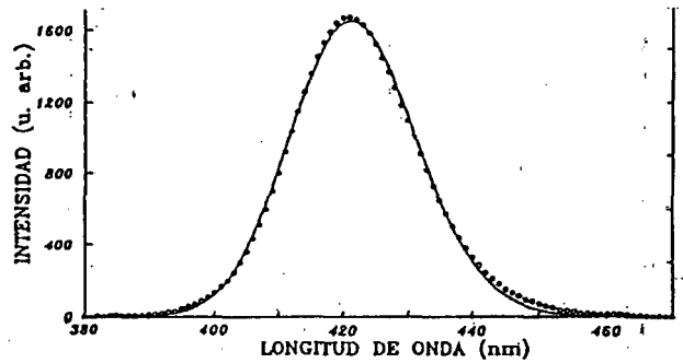
Fig. 3. Espectro de emisión del \text{Eu}^{2+} en KCl.
