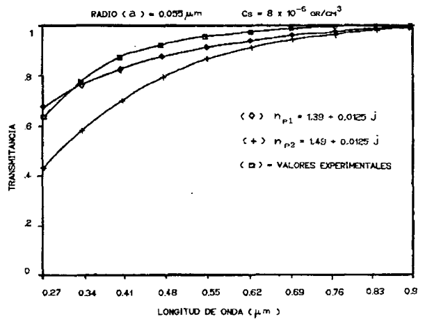
Fig. 7: Transmitancia de la muestra en función de la longitud de onda.
