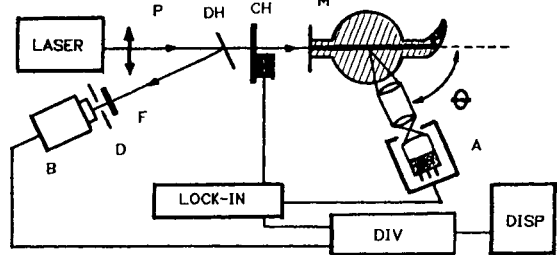
Fig. 1: Nefelómetro utilizado para medición de radio de partículas. Láser: He-Ne de 5 mW, no polarizado. DH: divisor de haz. P: polarizador. M: celda de vidrio con trampa de luz. F: filtro atenuador. D: diafragma. A: fotomultiplicador. B: fotodetector. DIV: divisor analógico. DISP: indicador numérico del cociente. CH: Chopper del Lockin.
