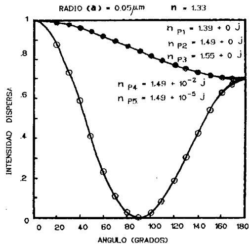
Fig. 2: Intensidad de luz dispersada en función del ángulo para tres índices de refracción cuya parte real es diferente ( n_{p1} , n_{p2} y n_{p3} ) y dos índices de refracción con distinta parte imaginaria ( n_{p4} y n_{p5} ). (o) luz incidente polarizada paralelamente al plano de observación; (•) luz incidente polarizada perpendicularmente.
