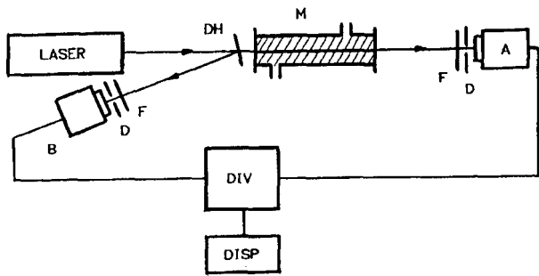
Fig. 3: Equipo utilizado para la medición de atenuación a una sola longitud de onda. Láser: He-Ne de 5 mW no polarizado. DH: divisor de haz. M: celda, longitud: 22,3 cm. F: filtro atenuador. D: diafragma. A: fotodetector para medir la intensidad de luz atenuada por la muestra. B: fotodetector para medir intensidad de referencia. DIV.: divisor analógico y convertor analógico-digital. DISP: indicador numérico del cociente.
