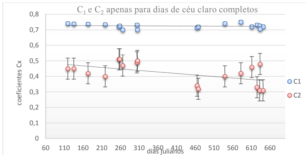
Figura 2. Valores dos coeficientes C_1 e C_2 obtidos para dias de céu claro nos anos de 2012 e 2013.
