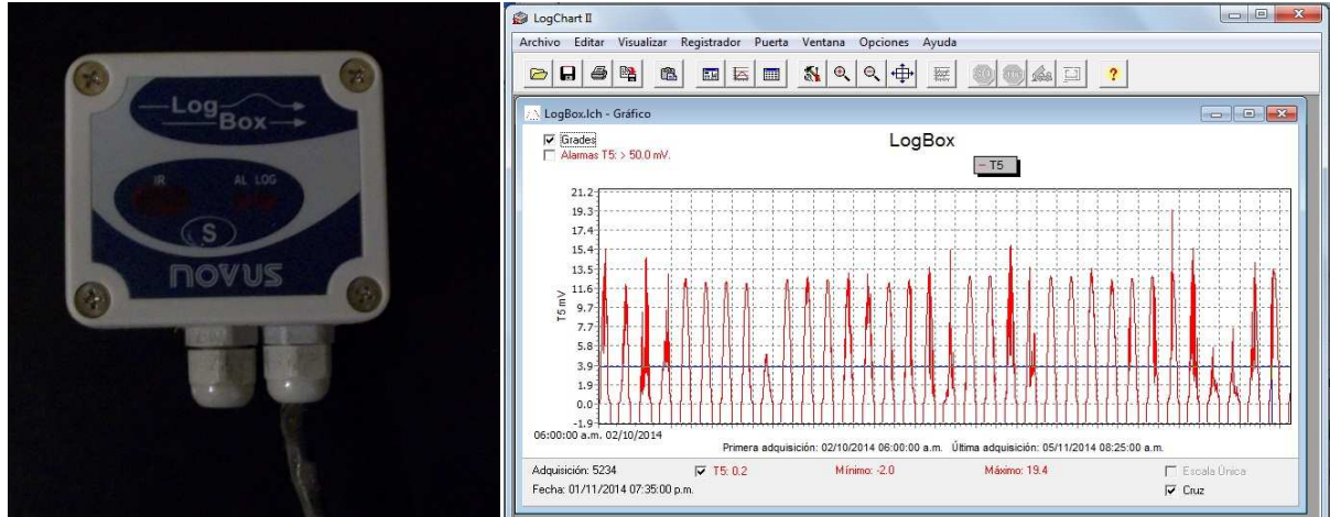
Fig. 2. LogBox - AA-32K-IP65 e Imagen generada por LogChart II, durante la descarga de datos.
