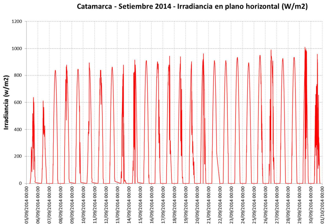
Figura 3: Irradiancia en plano horizontal – Septiembre de 2014
