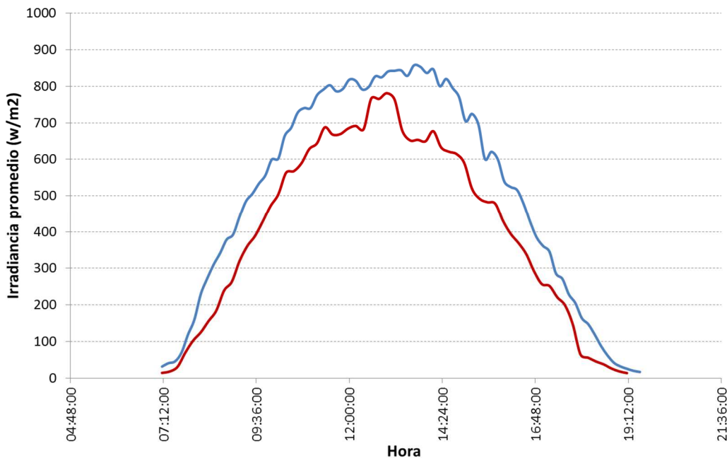
Figura 5: Curva comparativa de los días promedio (IDP) de Septiembre y Octubre de 2014
