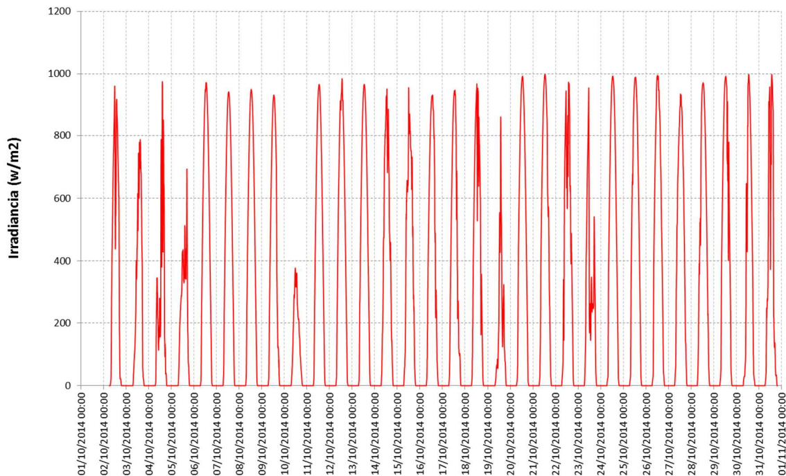
Figura 4: Irradiancia en plano horizontal – Octubre de 2014
