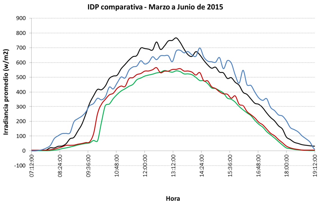
Figura 6: Curva comparativa de los días promedio (IDP) de Marzo a Junio de 2015
