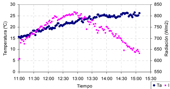
Figura 5: Datos ambientales del día de ensayo (22-jun.).
