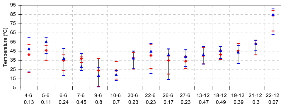
Figura 10: Temperatura de flujo a la salida del colector, por debajo y arriba del absorbedor.
