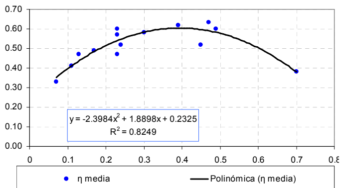
Figura 13: Curva de eficiencia versus caudal, \eta(m) , donde m está expresado en kg/s.
