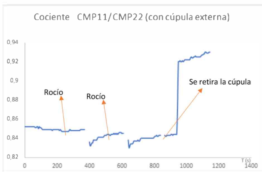
Figura 5: Efecto del rocío de gotas de agua sobre la cúpula adicional colocada sobre el CMP11. Nótese el rápido descenso del cociente de los voltajes y, cuando se retira la cúpula, el inmediato ascenso a los valores previos.
