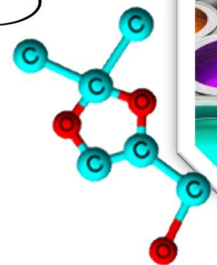
Solketal
