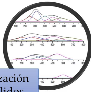
Solketal
