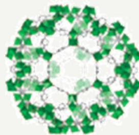
MIL-101 (X)
