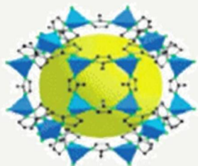
ZIF-8
