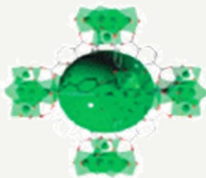
UiO-66
