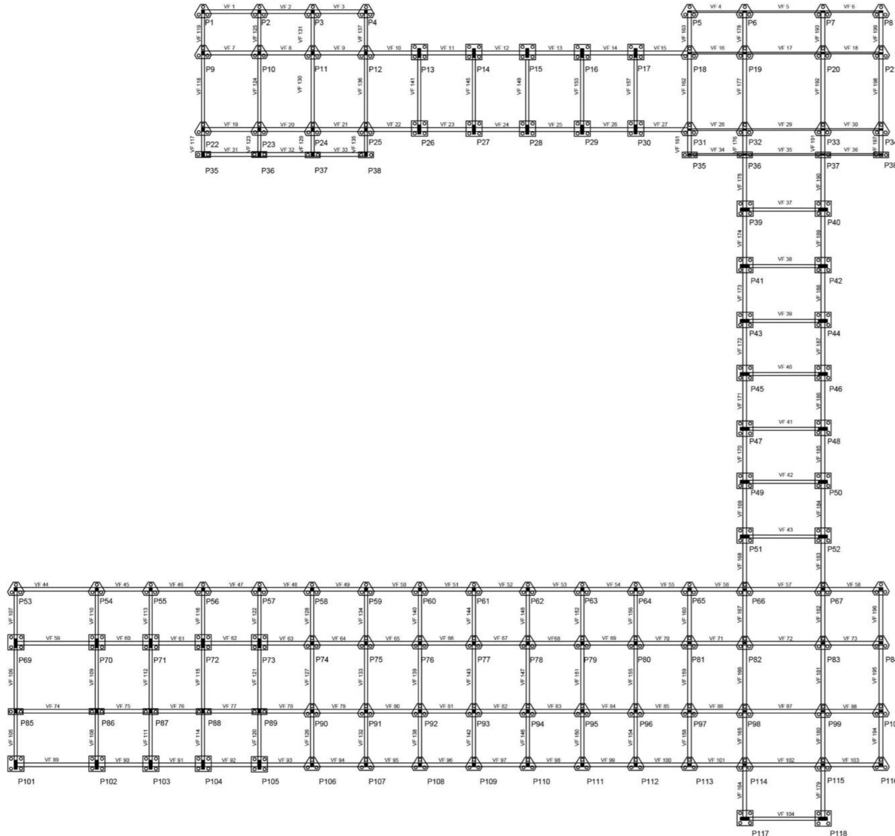
PLANTA DE FUNDACIONES
