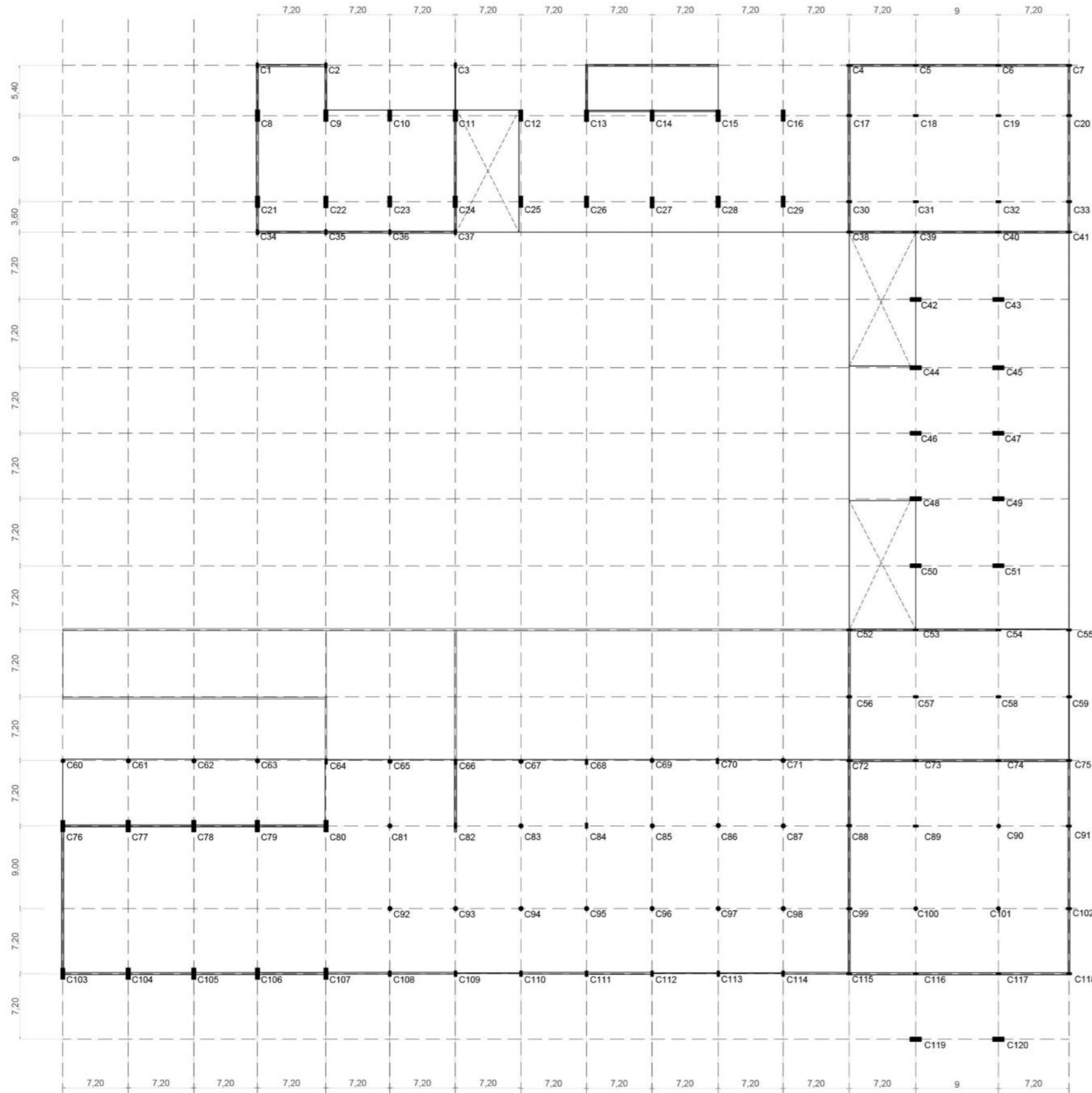
COLUMNAS SOBRE PB
