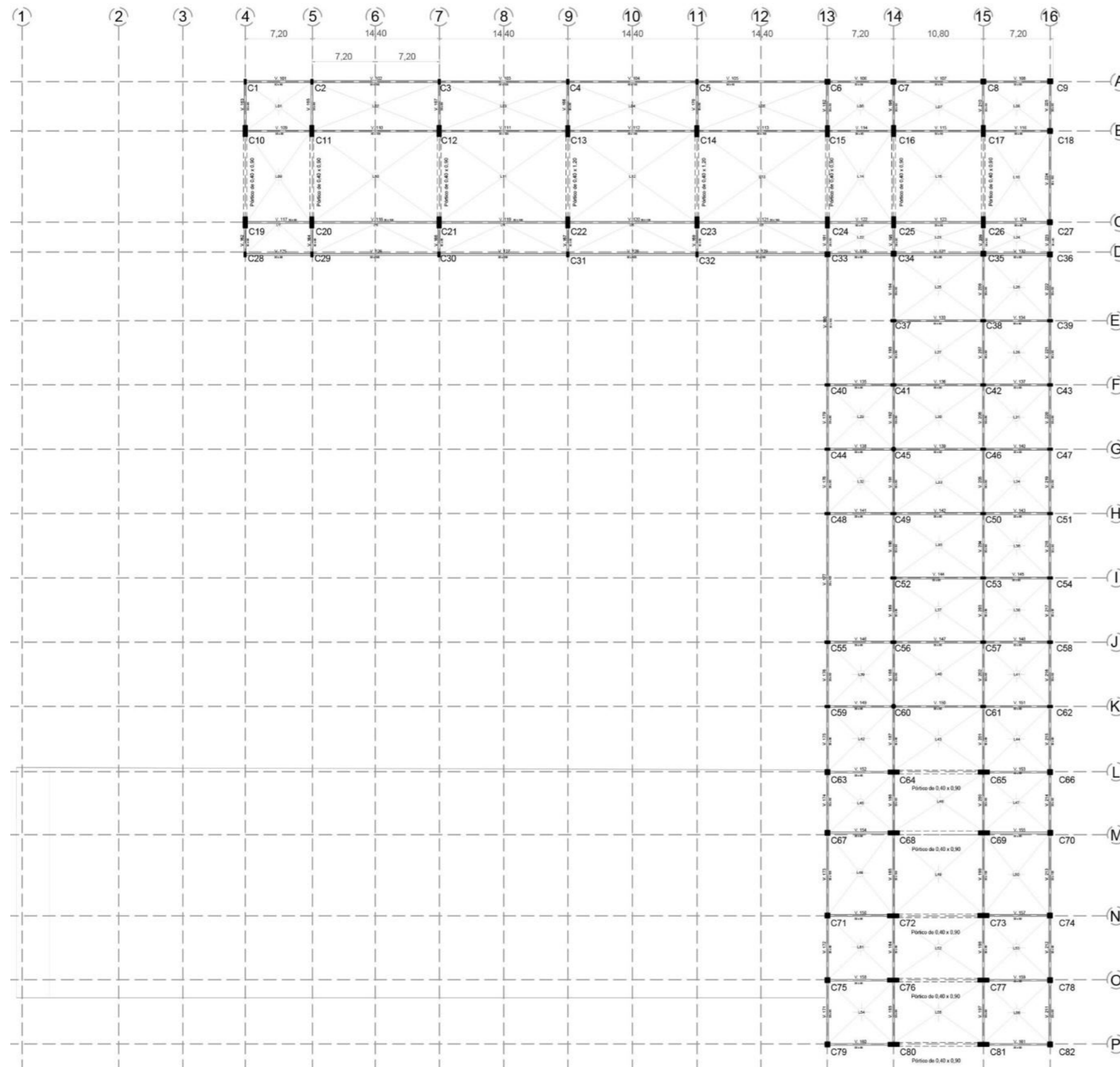
ESTRUCTURA SOBRE P1
