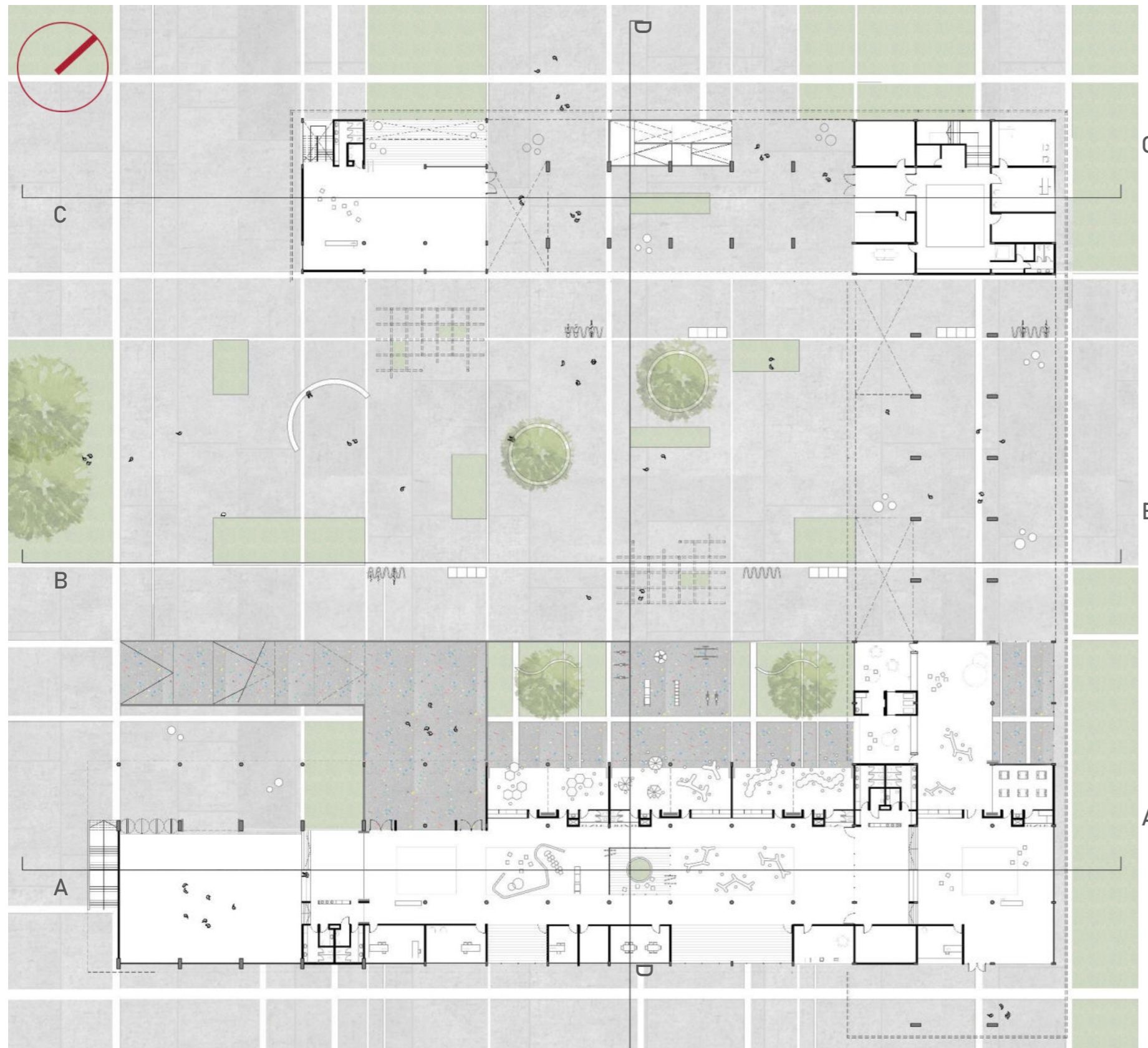
PLANTA BAJA ESC. 1 EN 100
