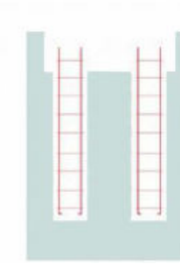
2 Colocación de armadura en p pilotes
