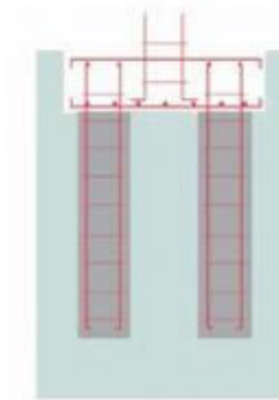
4 Colocación de armadura en cabezal
