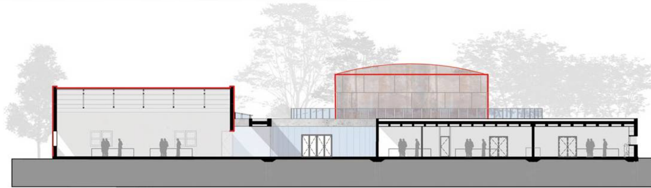
CORTE A-A
