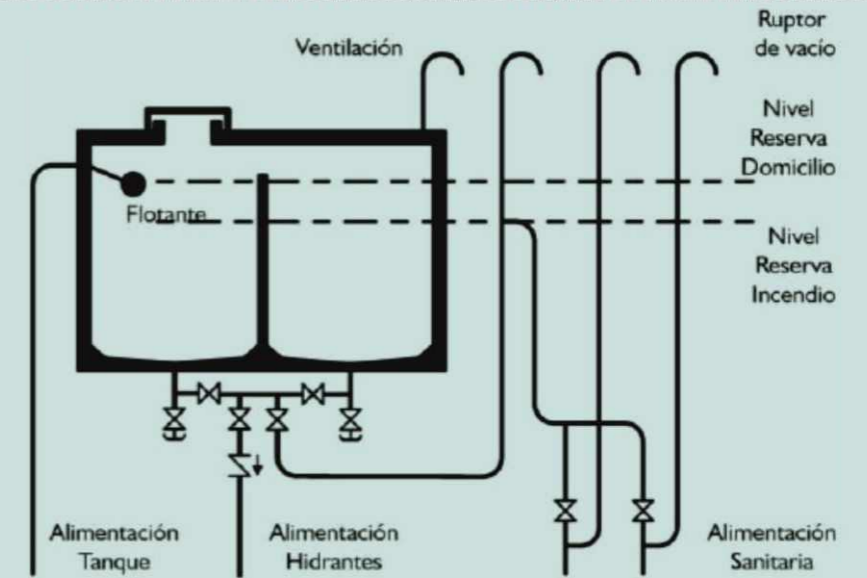
Esquema tanque de reserva
