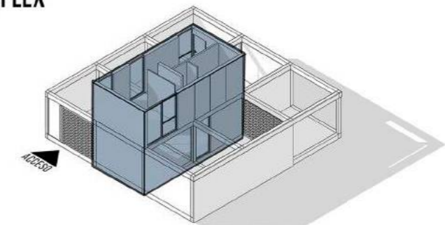
CÉLULA MÍNIMA (4 SUBMÓDULOS: 1 SOCIAL, 1 PRIVADO Y 2 NÚCLEOS)
