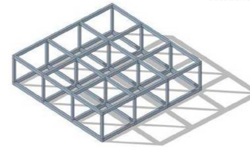
MÓDULO Y SUBMÓDULO CONFIGURADO EN GRILLA ESTRUCTURAL
