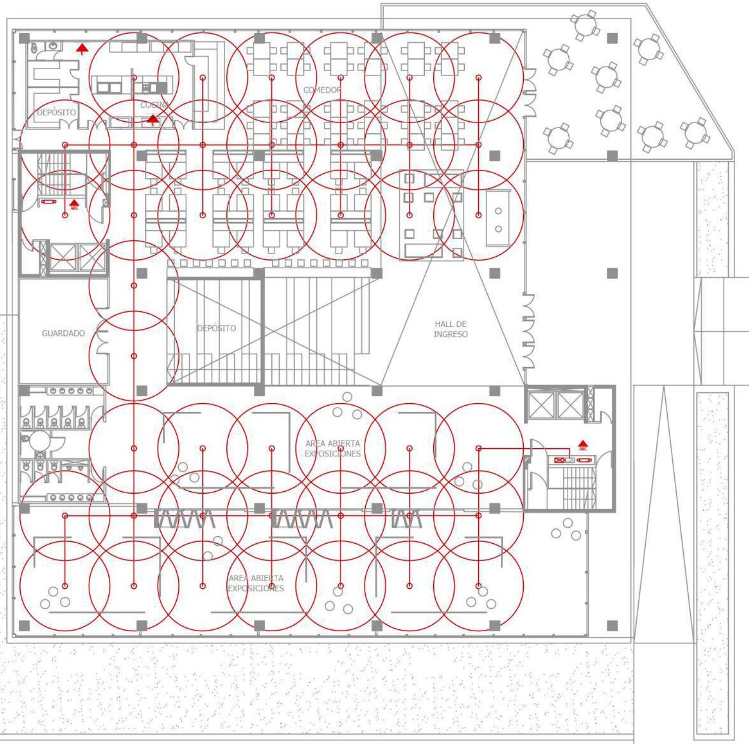
Tendido en planta baja área común
