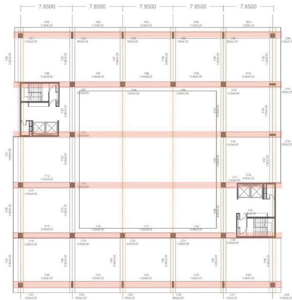
SISTEMA DE COLUMNAS Y FAJAS HºAº
