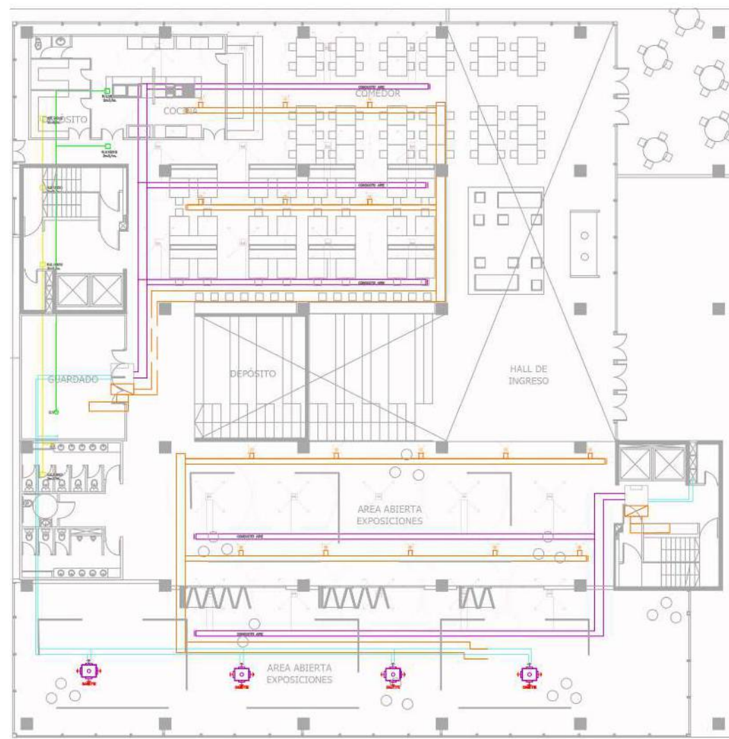
DISTRIBUCIÓN EN PB
