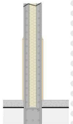
Detalle tabique
