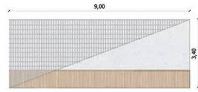
MURO 17 9,00m x 3,40m Cantidad: 6
