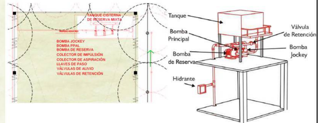
Esquema Tanque y bombas
