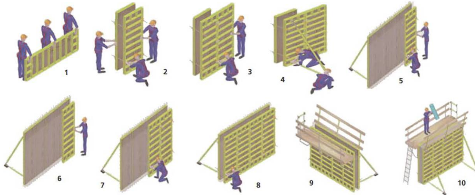
Esquema de armado de encofrados para un tabique de hormigón
