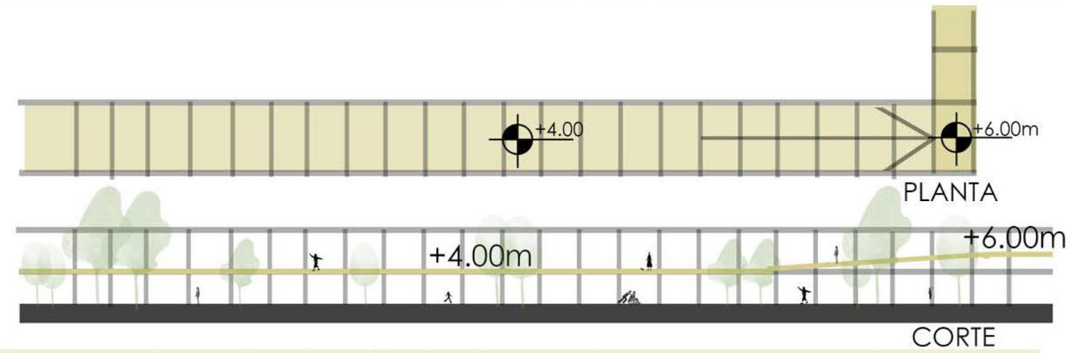
Conector longitudinal a nivel +4m con empalme a conector transversal
