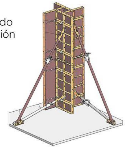
Esquema armado columna
