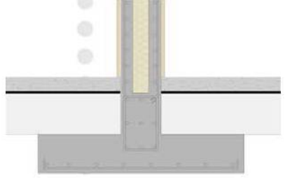
Zapata corrida y tabique de H°A°
