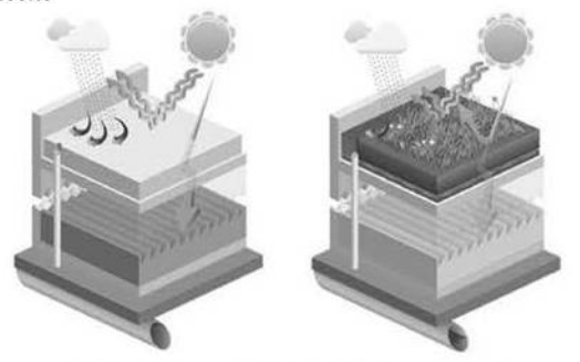
Esquema de diferencias entre una cubierta verde y una convencional
