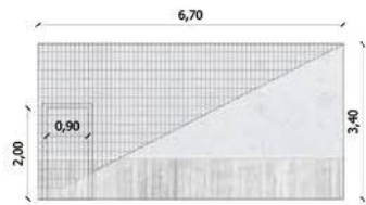
MURO 8 6,70 m x 3,40m Cantidad: 2 CON PUERTA 0,90m
