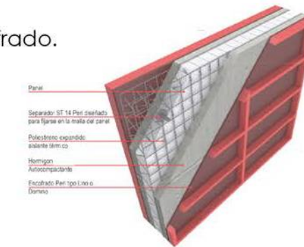
Esquema armado tabique y aislación
