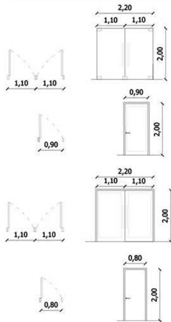
Puerta 1: doble puerta de vidrio templado
