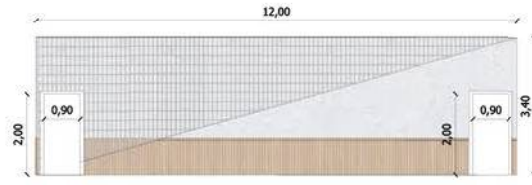
MURO 21 12,00 m x 3,40m Cantidad: 1 2 PUERTAS 0,90m
