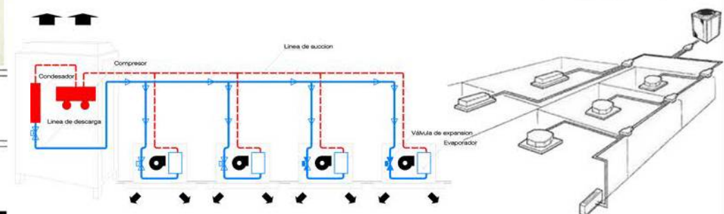
Esquema funcionamiento VRV
