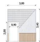
MURO 10 3,00m x 3,40m Cantidad: 3 CON PUERTA 0,90
