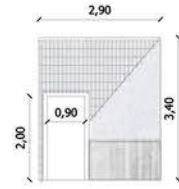
MURO 3 2,90m x 3,40m Cantidad: 4 CON PUERTA 0,90m
