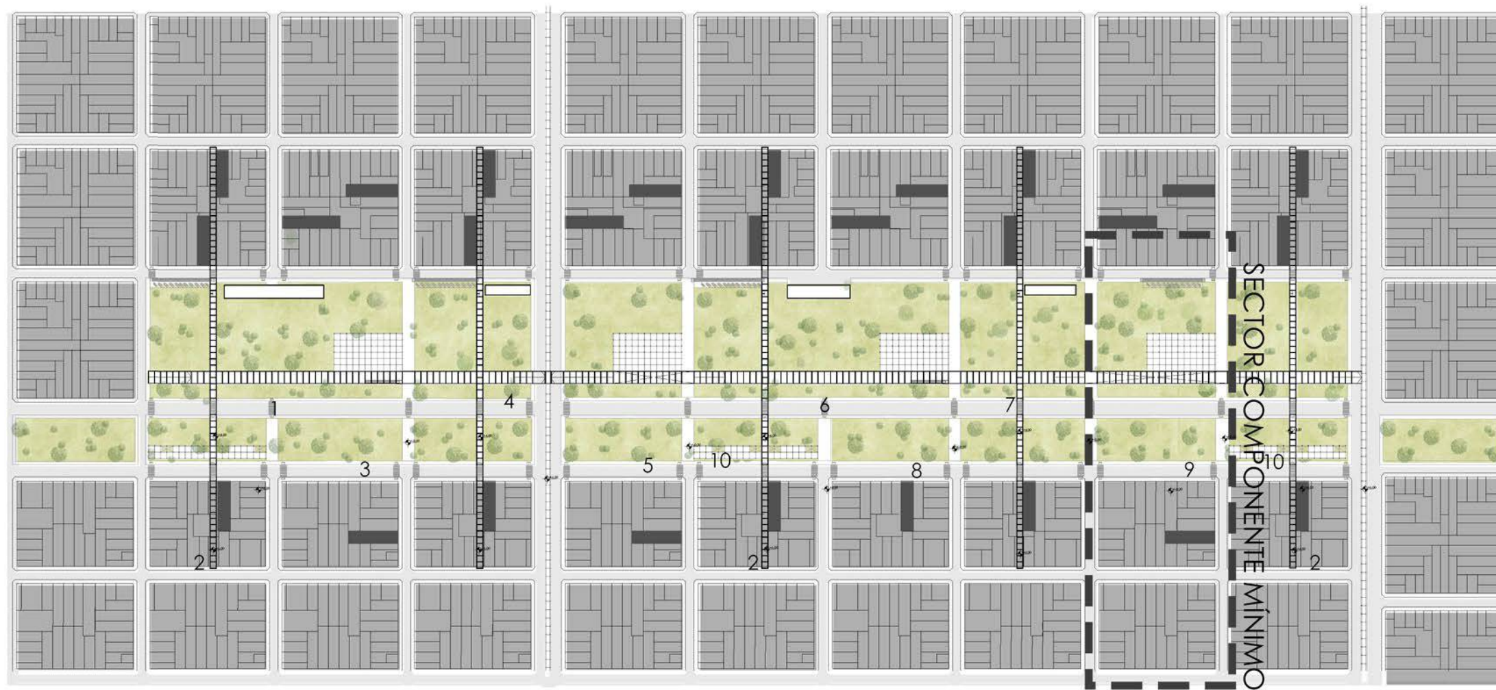
PLANTA MERIDIANO QUINTO
