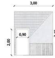
MURO 5 3,00m x 3,40m Cantidad: 2 CON PUERTA 0,90m
