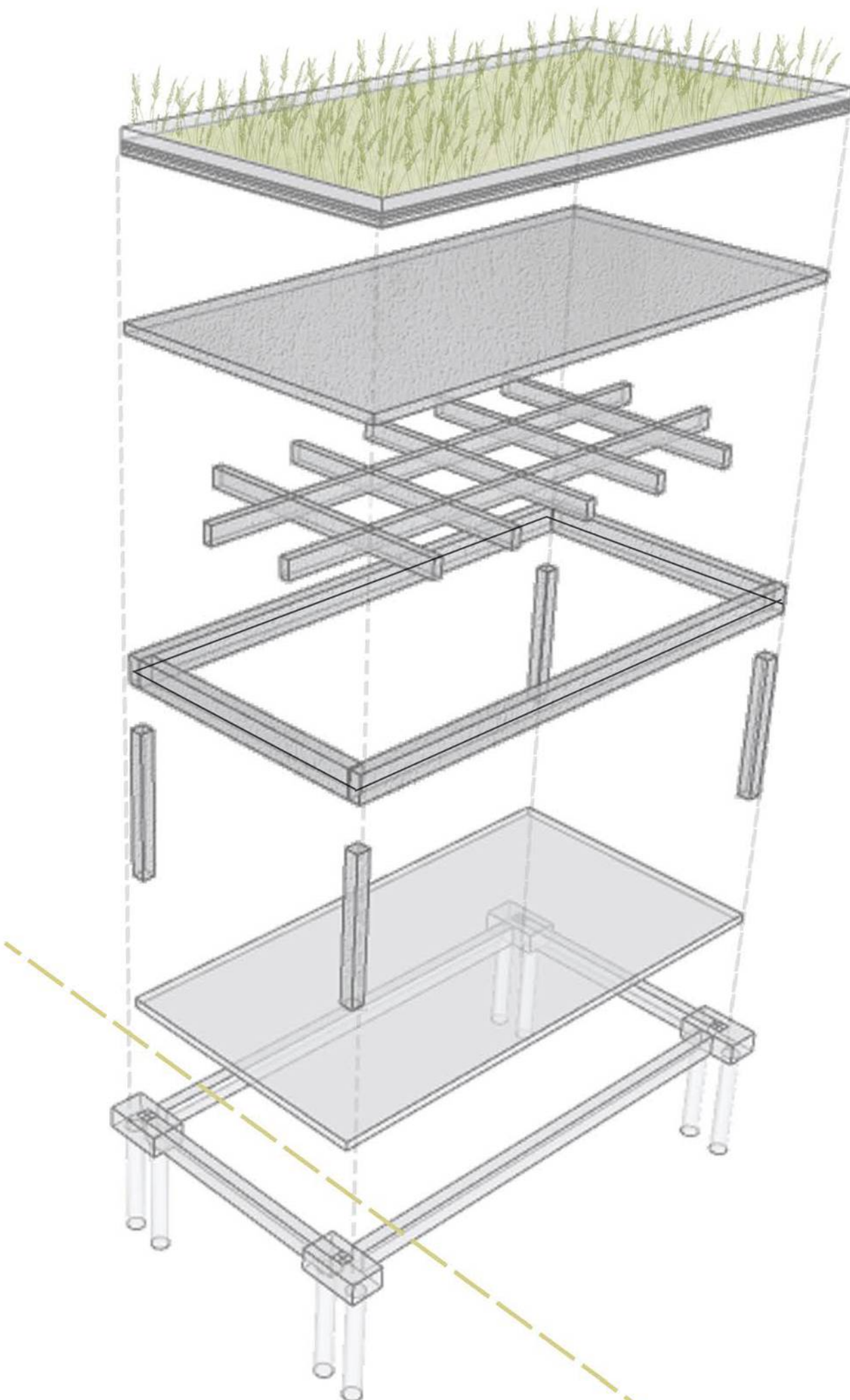
Despiece esquemático de sistemas Sostener-apoyar y cubrir
