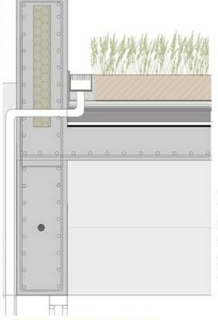
Esquema de diferencias entre una cubierta verde y una convencional
