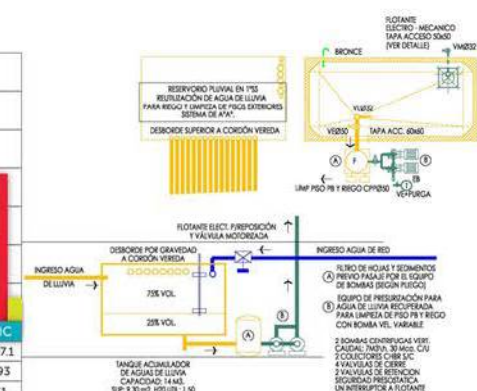
Esquema tanque de acumulación
