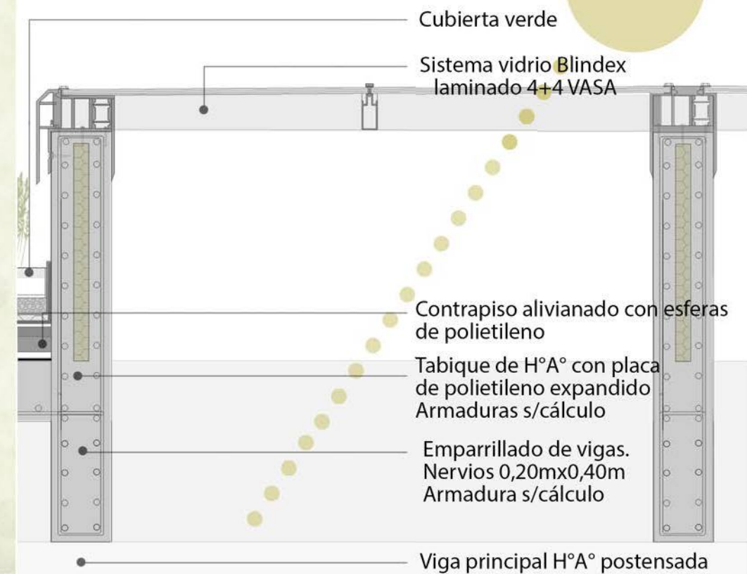
DETALE ESTRUCTURA LUCARNAS
