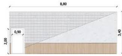
MURO 16 8,80m x 3,40m Cantidad: 2 1 PUERTA 0,90m
