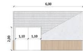
MURO 13 6,00m x 3,40m Cantidad: 4 1 PUERTA 2,20m
