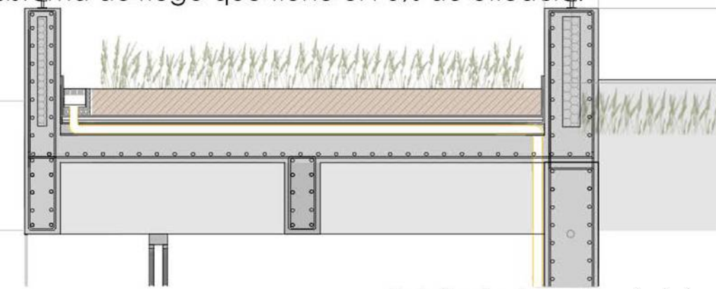
Detalle de desagües pluviales
