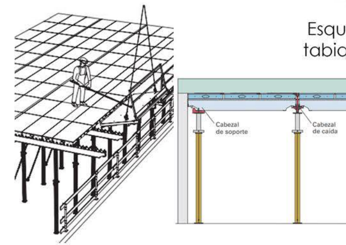
Esquema armado losa
