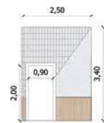
MURO 4 2,50m x 3,40m Cantidad: 2 1 PUERTA 0,90m
