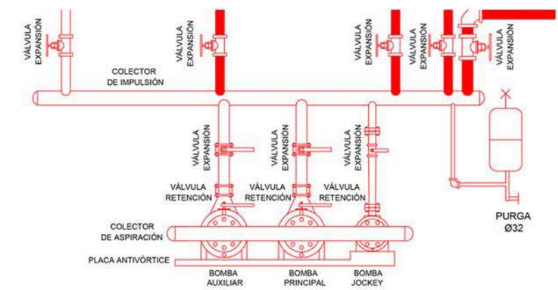
Detalle Bombas
