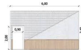
MURO 12 6,00m x 3,40m Cantidad: 4 1 PUERTA 0,90m
