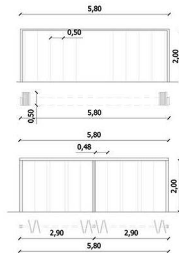
Paneles corredizos SUM y Auditorio
