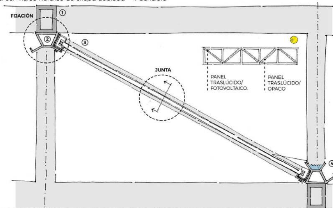
PANEL TRASLÚCIDO
