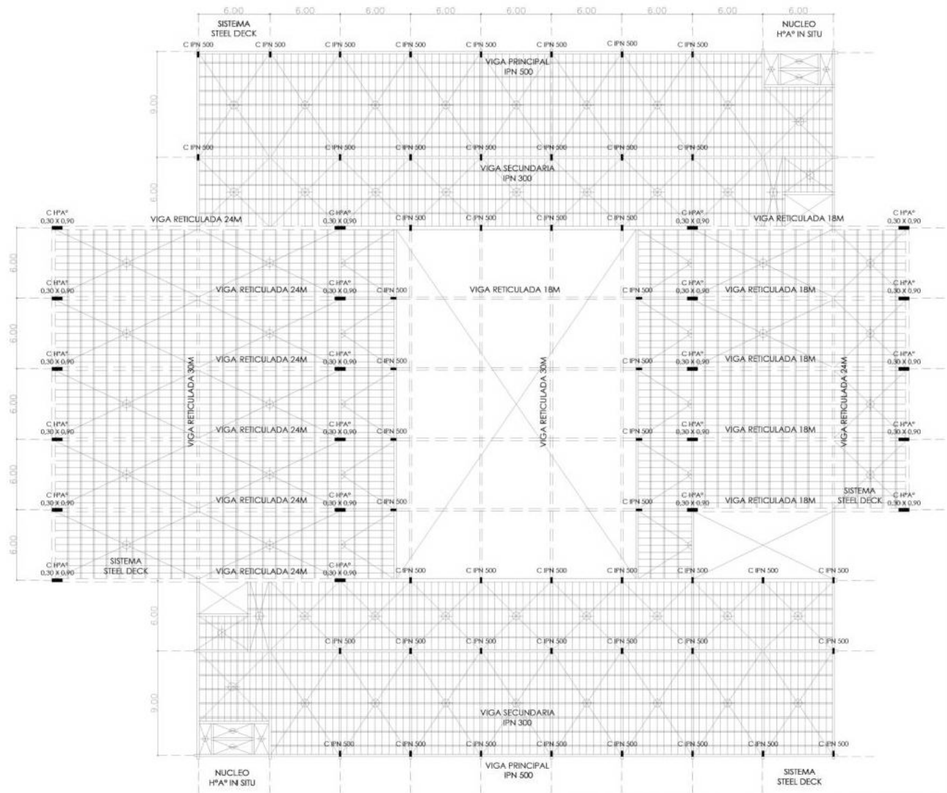
PLANTA ESTRUCTURAL +5 ESC 1 300
