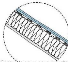
PANEL FOTOVOLTAICO
