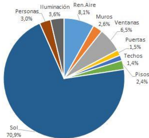
Figura 8: Aportes térmicos discriminados. Situación mejorada verano.
