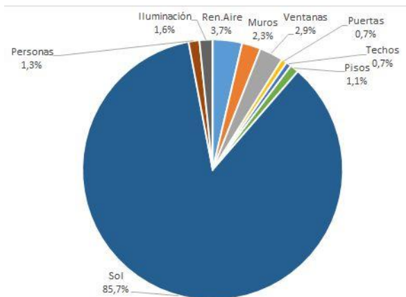
Figura 6: Aportes térmicos discriminados. Situación original verano.
