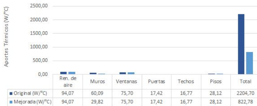
Figura 9: Comparación de edificio original y mejorado. Situación verano.
