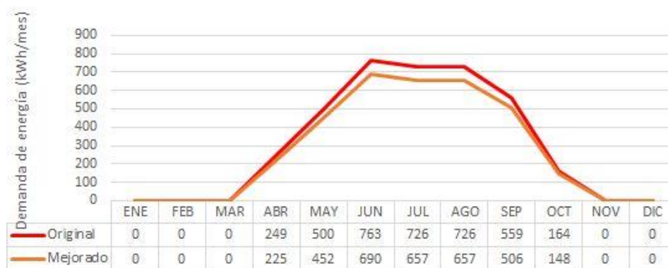
Figura 5: Comparación entre versión original y mejorada mensual
