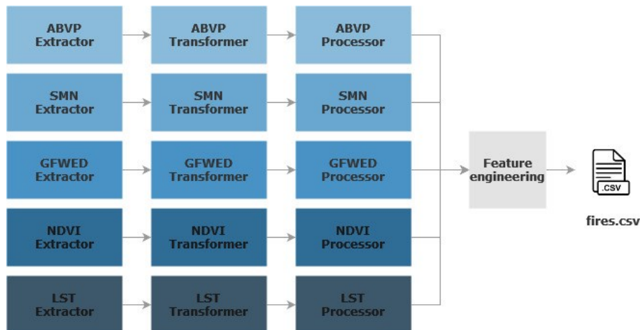
Fig. 1. Arquitectura conceptual del pipeline de datos.
