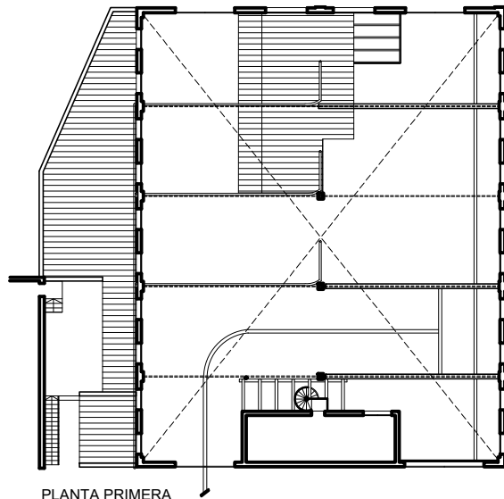
PLANTA PRIMERA
