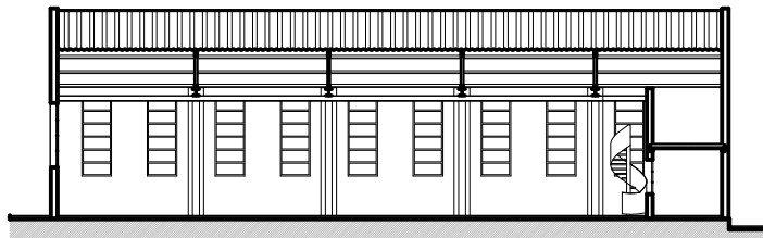
CORTE LONGITUDINAL C
