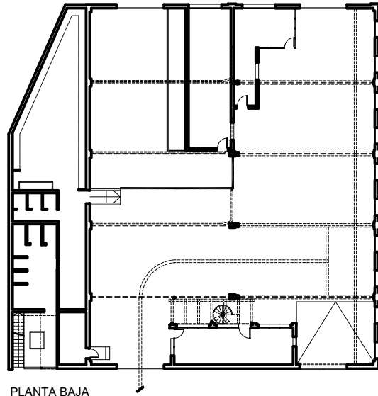
PLANTA BAJA
