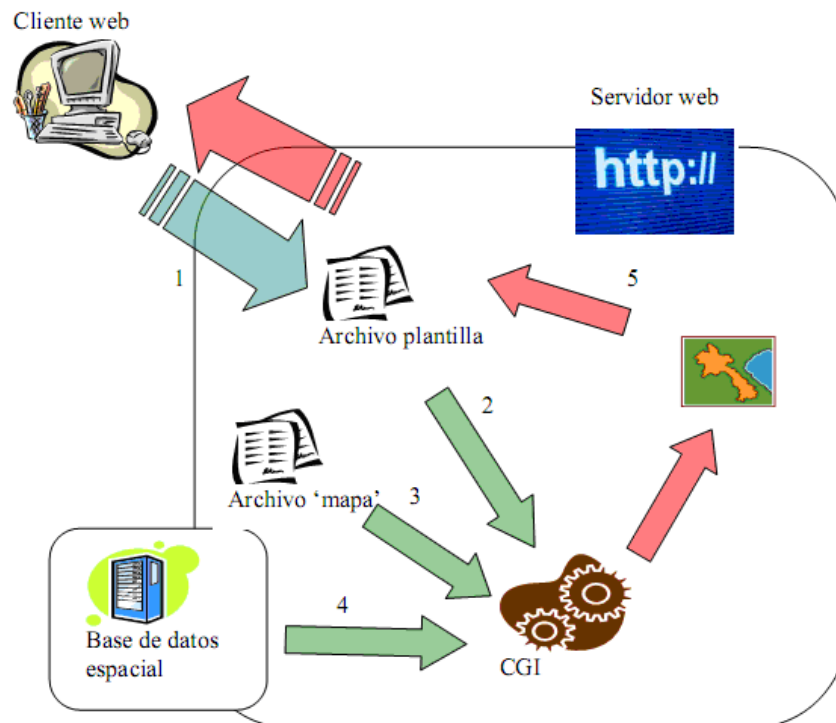
Fig. 1 Esquema de Funcionamiento de MapServer
