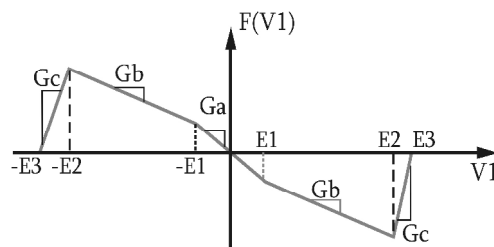
Fig. 2. Característica del elemento no lineal denominado Diodo de Chua. Presenta pendientes negativas G_a y G_b hasta el punto de quiebre E2 dependiente del voltaje de saturación de los amplificadores operacionales que conforman el Diodo de Chua.
