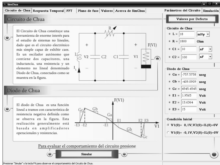
Fig. 4. Inicio de SimChua. Se puede observar una breve descripción del circuito de Chua y los valores que el programa le asigna por defecto al modelo para poder comenzar a estudiarlo.
