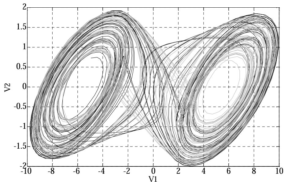
Fig. 3. Scroll Doble para R=1881\Omega . Los demás parámetros responden a lo descrito en [9]. En negro se observa el comportamiento caótico medido en el laboratorio sobre el circuito de Chua, en gris se observa la dinámica que entrega SimChua; ambos muy similares.
