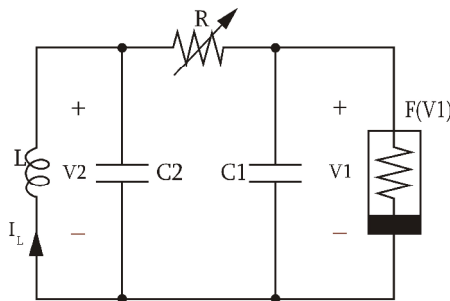
Fig. 1. Esquema de conexión del Circuito de Chua. El mismo está conformado por dos capacitores, una inductancia, una resistencia y un elemento no lineal conocido como Diodo de Chua.
