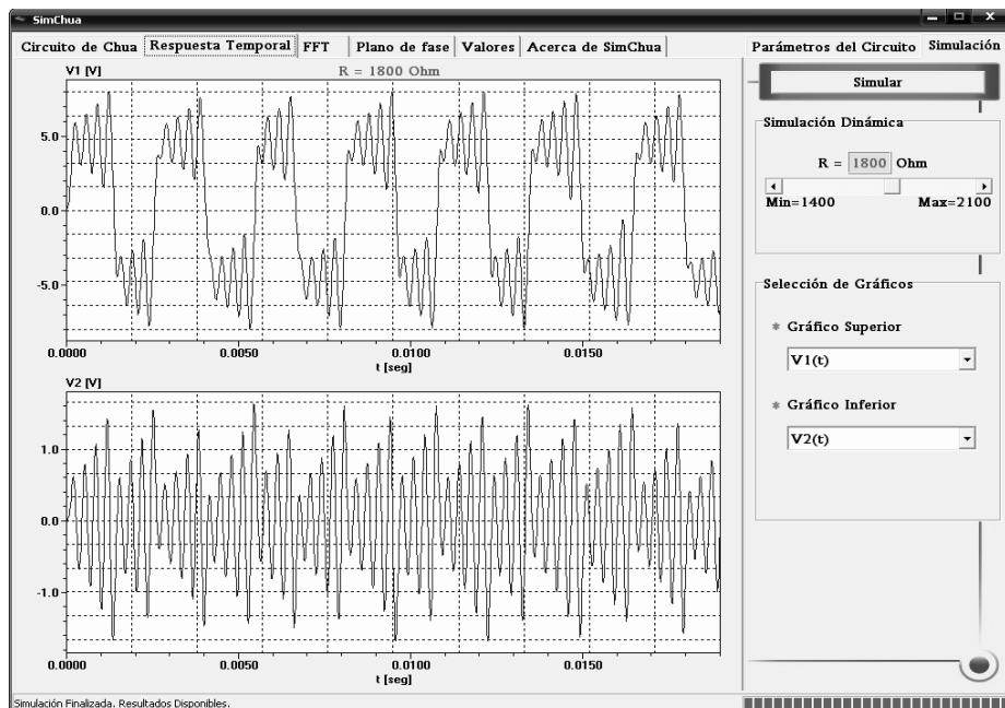
Fig. 5. Resultado de la simulación del sistema para los valores por defecto. Desde la pestaña Simulación podemos configurar qué respuesta temporal mostrar, o acceder a la Simulación Dinámica.
