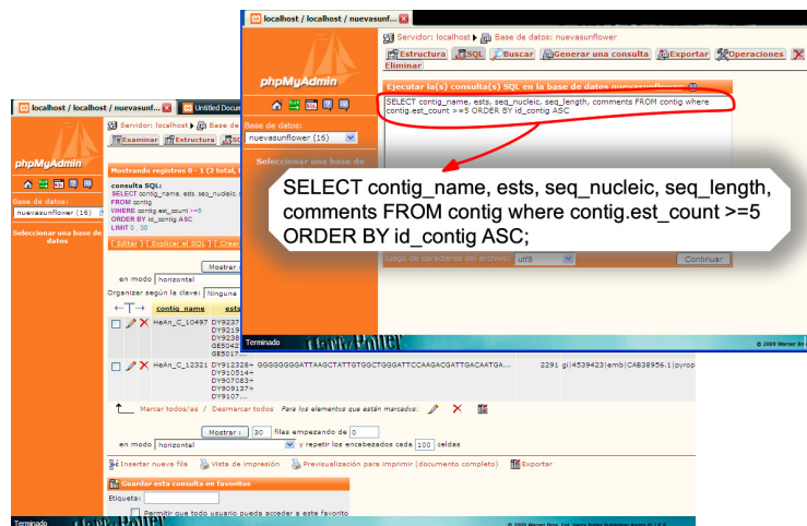
Fig. 1 Interfaz clásica de una consulta en lenguaje SQL
