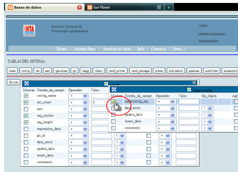
Fig 3-a Interfaz de consulta visual de la SfGD
