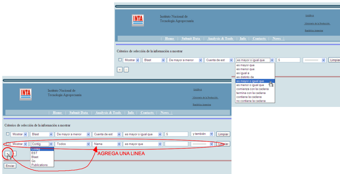
Fig. 4 La misma consulta de la Fig. 3-b se reduce a seleccionar en una línea las opciones adecuadas. Se pueden agregar más condiciones en nuevas líneas.
