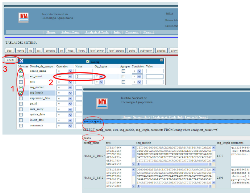
Fig 3-b Consulta por formulario: “mostrar todos los contig con 5 o más EST”
