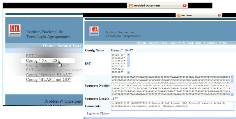
Fig. 2 Consulta rutinaria: “mostrar todos los contig con 5 o más EST”
