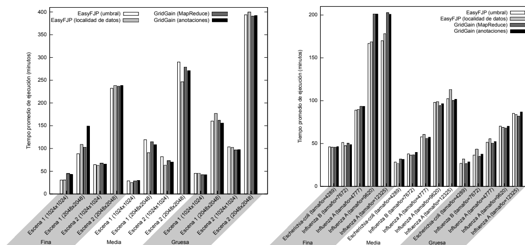
Figura 3: Tiempo promedio de ejecución para las aplicaciones
