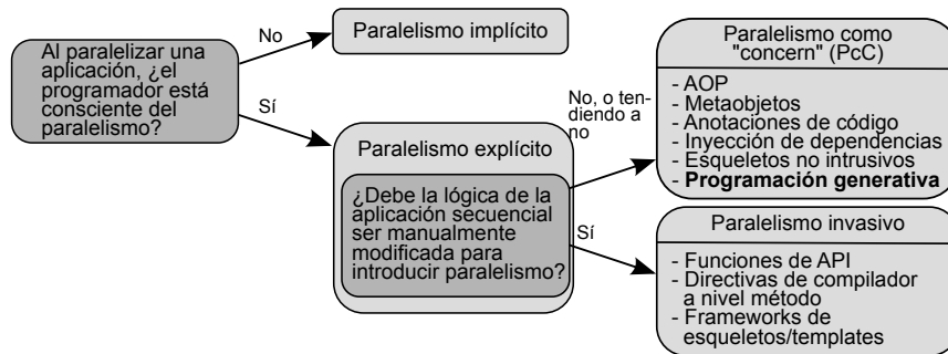
Figura 1: Taxonomía de las formas de paralelizar aplicaciones en Java
