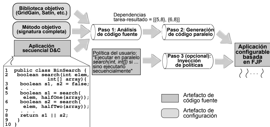
Figura 2: Vista general del proceso de paralelización de EasyFJP
