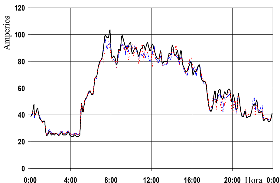
Figura 8. Consumo de corriente por fase a lo largo de 24 hs.
