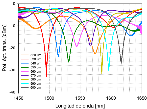
Figura 14. Sintonización del pico de atenuación de una LPG al cambiar el periodo de la red.
