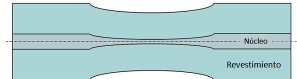
Figura 4. Esquema de un \mu - taper .
