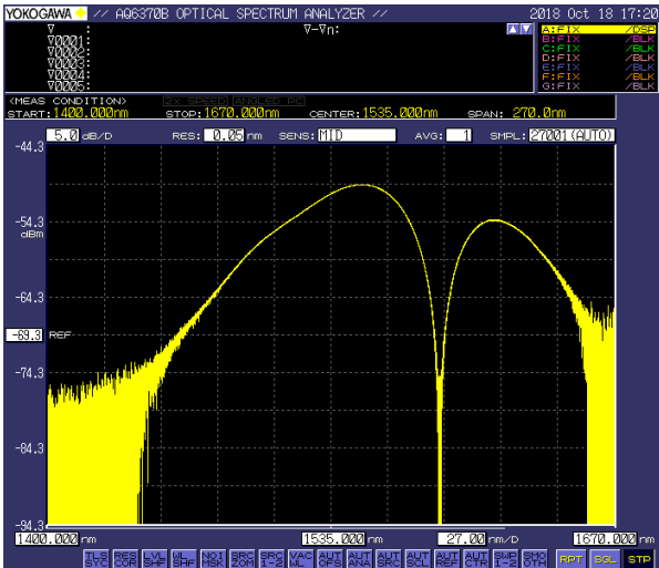
Figura 11. Captura de pantalla del instrumento analizador de espectros.
