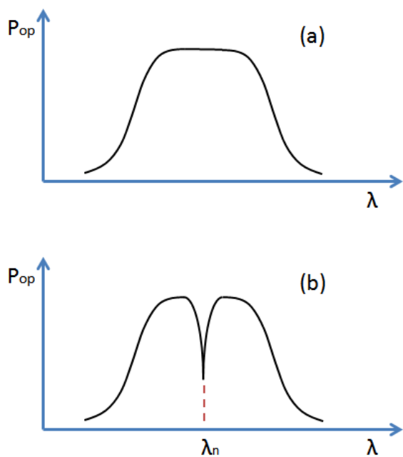
Figura 3. Espectro de la radiación luminosa: (a) antes y (b) después de atravesar la LPG.
