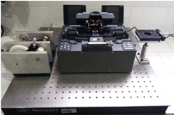
Figura 9. Arreglo experimental de generación de LPGs.
