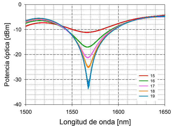
Figura 13. Ciclo de crecimiento del pico de atenuación durante la fabricación de una LPG.
