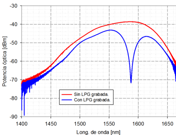
Figura 12. Respuesta a la transmisión de una fibra con y sin LPG grabada.
