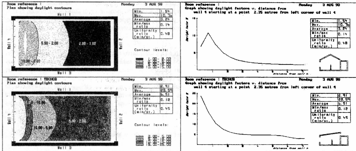
Figura 4. Comparación de distribución de la iluminación natural en dos casos. (Techo "A", avent. 25%, clara y Techo "C", avent. 50%, clara). Malla de puntos 15 x 15.
