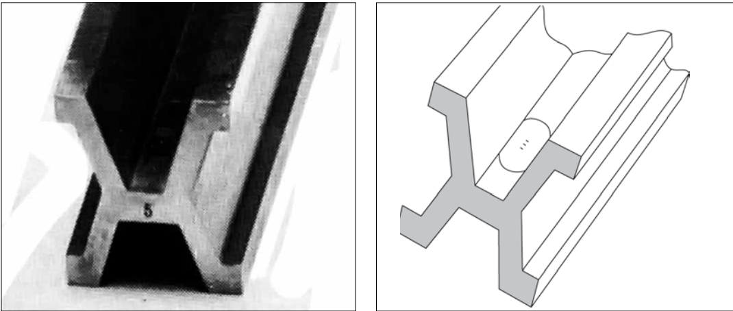
Fig. 12. Fotografía del extremo de identificación de la barra en X N.º 5 Fig. 13. Dibujo del extremo de una barra en X y los tres trazos grabados. La distancia entre los trazos medios de los extremos definen el metro.
