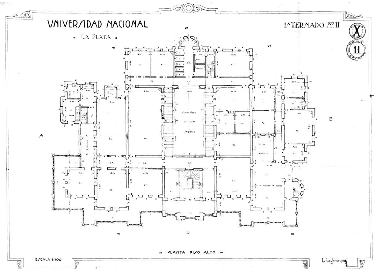
PLANTA PRIMERA
