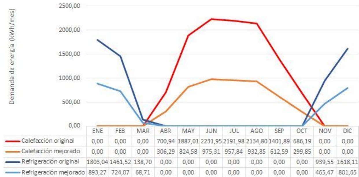
Figura 1: Comparación de demandas de energía en climatización mensual original y con mejoras.
