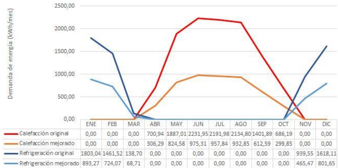
Figura 11: Comparación anual caso: Defensa Civil, Neuquén. Neuquén.
