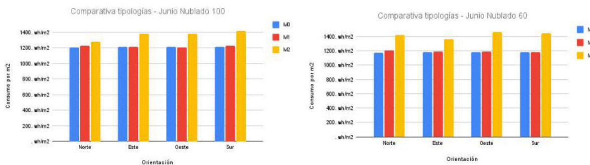
Figuras 16 y 17. Gráficos comparativos demanda energética de calefacción por m^2 habitable. Día de invierno nublado superficie vidriada 60% y 100%. M0, M1, M2. Fuente: Elaboración propia del equipo.
