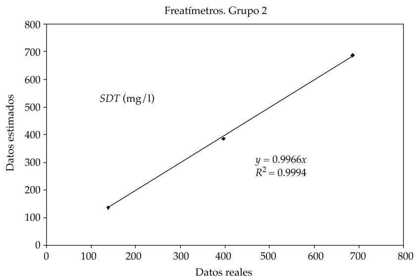
Figura 5. Relación entre valores reales y estimados por modelación matemática. Freatímetros, grupo 2.
