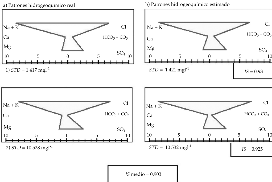
Figura 6. Comparación entre patrones hidrogeoquímicos y STD de datos reales a) y estimados b) por modelación hidrogeoquímica (modelo y = a_1x + a_2x^2 ). Muestras: 1) núm. 24 y 2) núm. 4 (pozos, grupo 4). Índice de similitud (IS).
