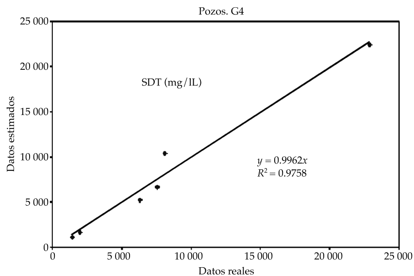
Figura 7. Relación entre valores reales y estimados por modelación matemática de STD; Pozos, grupo 4.
