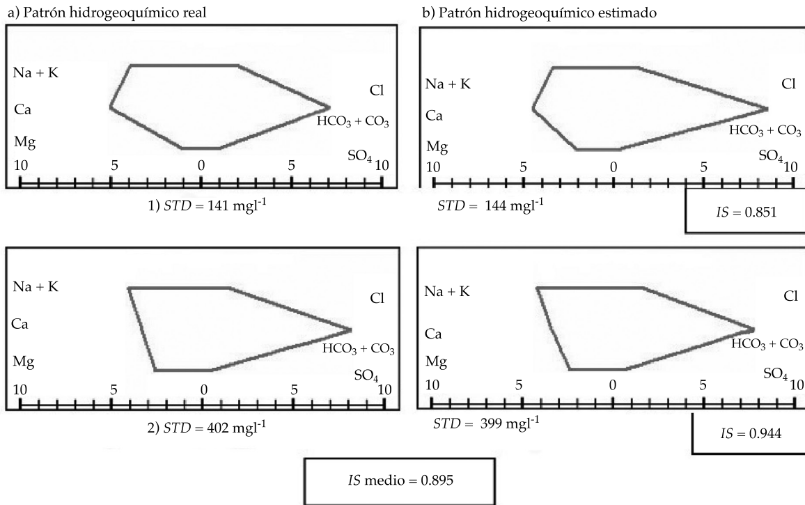
Figura 4. Comparación entre patrones hidrogeoquímicos y STD de valores reales a) y estimados b) por modelación hidrogeoquímica (modelo y = a_1x + a_2x^2 ). Muestras 1) núm. 10 y 2) núm. 17 (freatímetros, grupos 1 y 2, respectivamente). Índice de similitud (IS).
