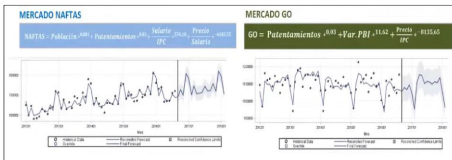
Fig. 2. Fórmulas predictivas tradicionales (YPF – 2020). Sobre el eje x se detalla la fecha (AñoDíaMes: 201201, 201301, etc), El eje y detalla el volumen de venta del combustible en m3, las líneas anteriores a la franja de pronóstico (zona de intervalo de confianza) son ajustes por gráfico de líneas sobre los valores de ventas históricas para el período en cuestión. Las variables que intervienen en las fórmulas siguen los formatos teóricos típicos [5]. La imagen fue generada por la empresa YPF.
