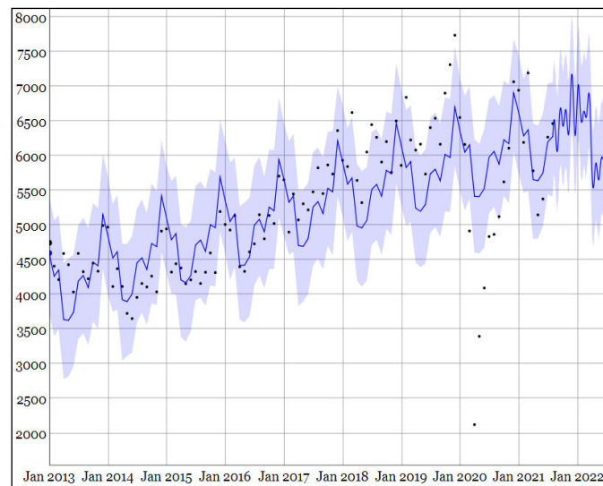
Fig. 10 – Pronóstico con herramienta Prophet de R (línea sólida azul) y ventas reales de Nafta. Los puntos representan los valores promedios por día sobre el total del territorio argentino graficados en m 3 . En el eje x la denominación “Jan” corresponde a la expresión anglosajona del mes de “Enero”. La herramienta Prophet es útil a nivel visual, y no sigue la modelización algebraica final que hemos propuesto. (Fuente: Elaboración propia, versión dinámica en [8] apartado “Estimaciones de demanda”, 2.1 “Naftas”).
