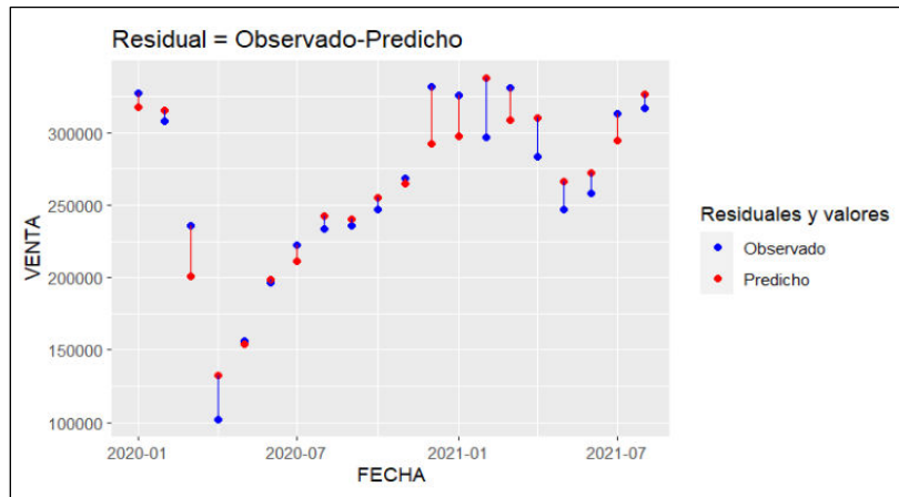
Fig. 15 – Gráfico de ventas mensuales de Nafta (medidos en m 3 ) desde datos abiertos oficiales de estaciones de servicio en el territorio nacional, y valor estimado por la fórmula pronóstico. Los segmentos en azul corresponden a la satisfacción de la demanda (la predicción supera a la venta real). (Fuente: Elaboración propia).
