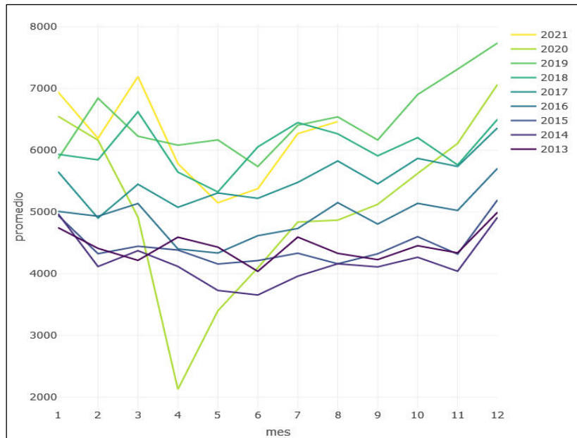
Fig. 6 – Venta sólo del combustible Nafta en Argentina 2013-2021, los valores graficados corresponden al promedio mensual (meses calendario 1 a 12) con unidad de medida m^3/10^2 [6]. (Fuente: Elaboración propia, versión dinámica en [8], apartado 2 “Estimaciones de Demanda”).
