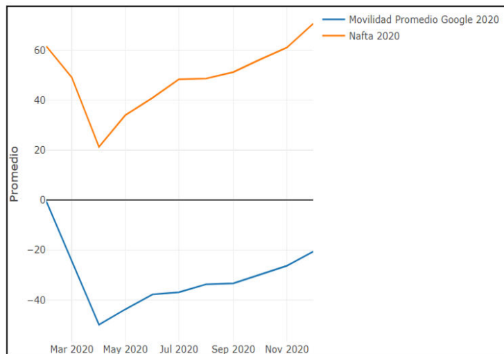
Fig. 12 – Comportamiento de la Movilidad promedio Google y la demanda de Nafta 2020. Los valores de la movilidad Google están expresados en variación porcentual (promedio de las 6 categorías destino informadas por Google) y los valores de la Nafta en promedio mensual sobre el territorio argentino en m^3/10^4 . (Fuente: Elaboración propia, versión dinámica en [8], apartado 3.1 -observación: leyenda corregida según fe de erratas en repositorio de origen propio-).
