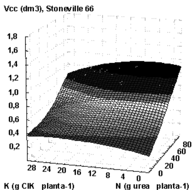
Figura 7. Crecimiento en volumen de leño con corteza (Vcc) del clon Stoneville 66 ante el aporte de distintas dosis y combinaciones de N y K, Ensayo N° 2 (2001-2002).
