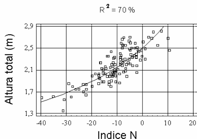
Figura 9. Asociación entre la respuesta de crecimiento en altura y el índice de N calculado por DRIS a partir de muestras de hojas en las parcelas de Stoneville 66 en la temporada 2000-2001.
