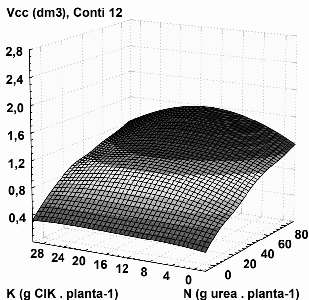
Figura 6. Crecimiento en volumen de leño con corteza (Vcc) del clon Conti 12 ante el aporte de distintas dosis y combinaciones de N y K, Ensayo N° 2 (2001-2002).
